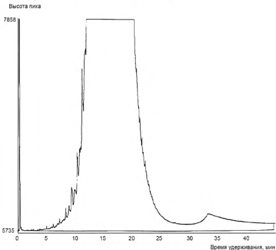
Рисунок 2 – Определение базовой линии образца моторного масла
