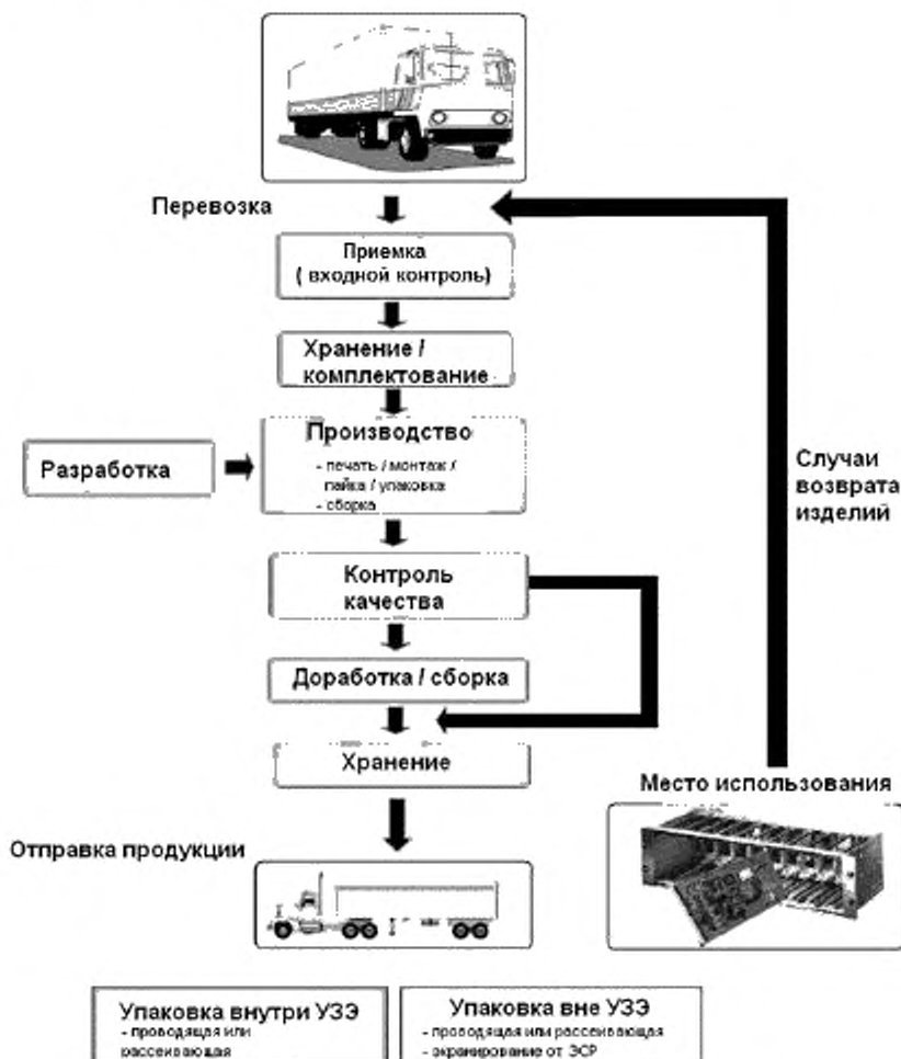
Рисунок А1 – Применение ЭСР защитной упаковки
