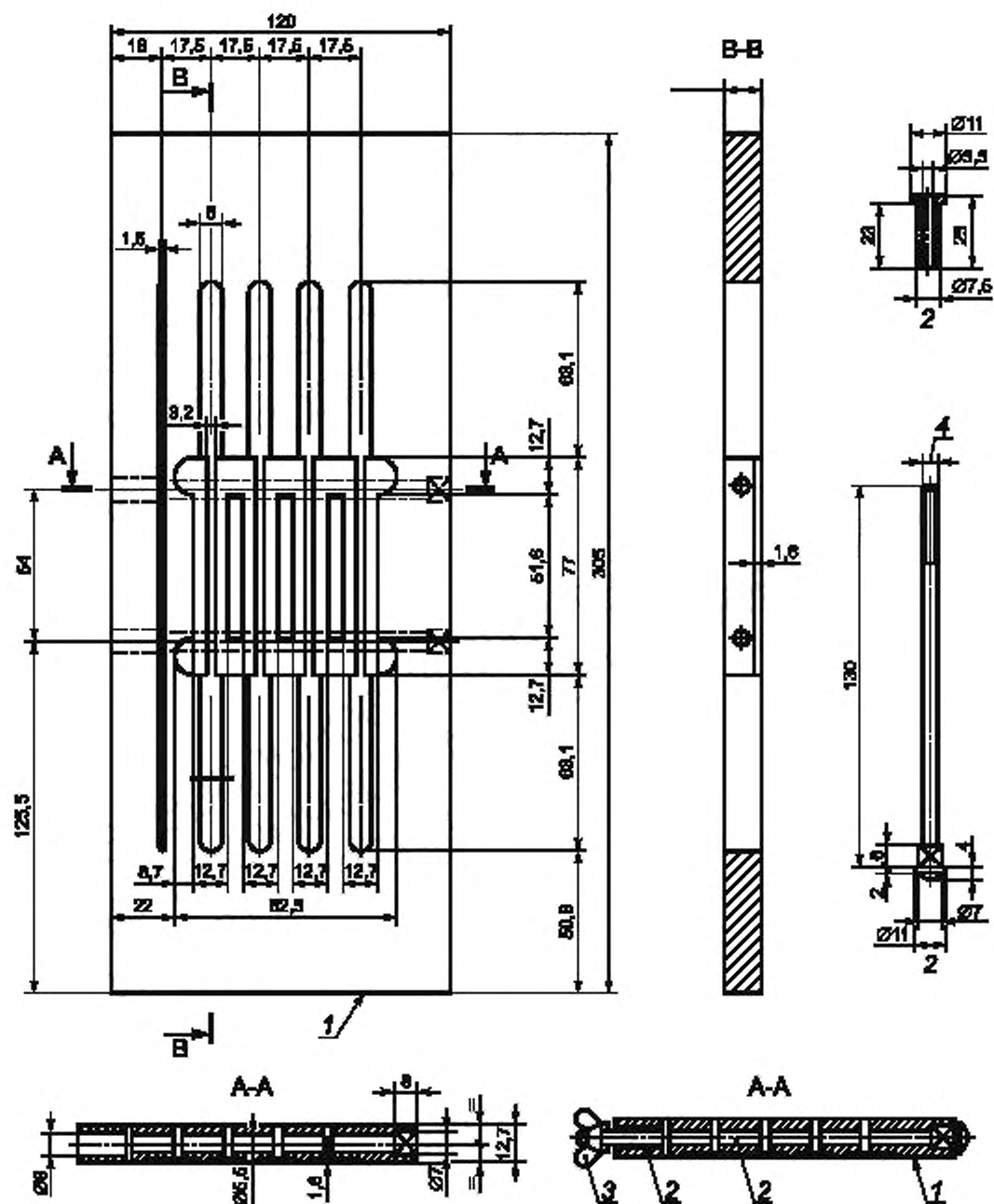
Рисунок X1.2 — Зажимное приспособление для нескольких пластинок
