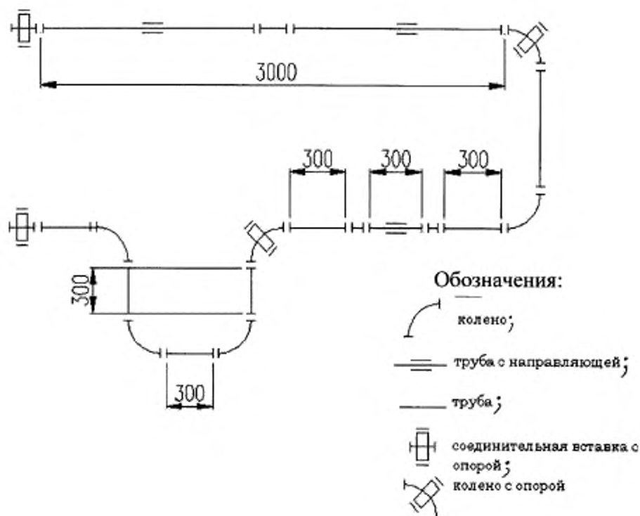
Рисунок Ж.1 — Испытательный образец для систем с трубами диаметром \leq 64 мм
