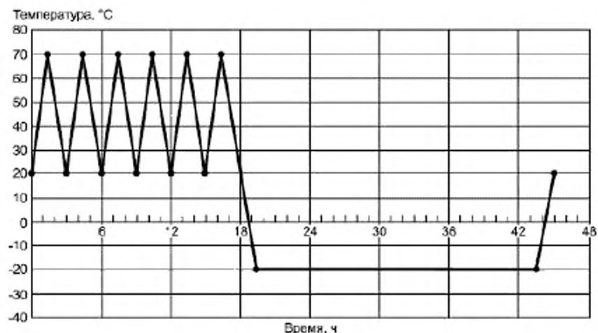
Рисунок Л.2 – Продолжительность циклов
