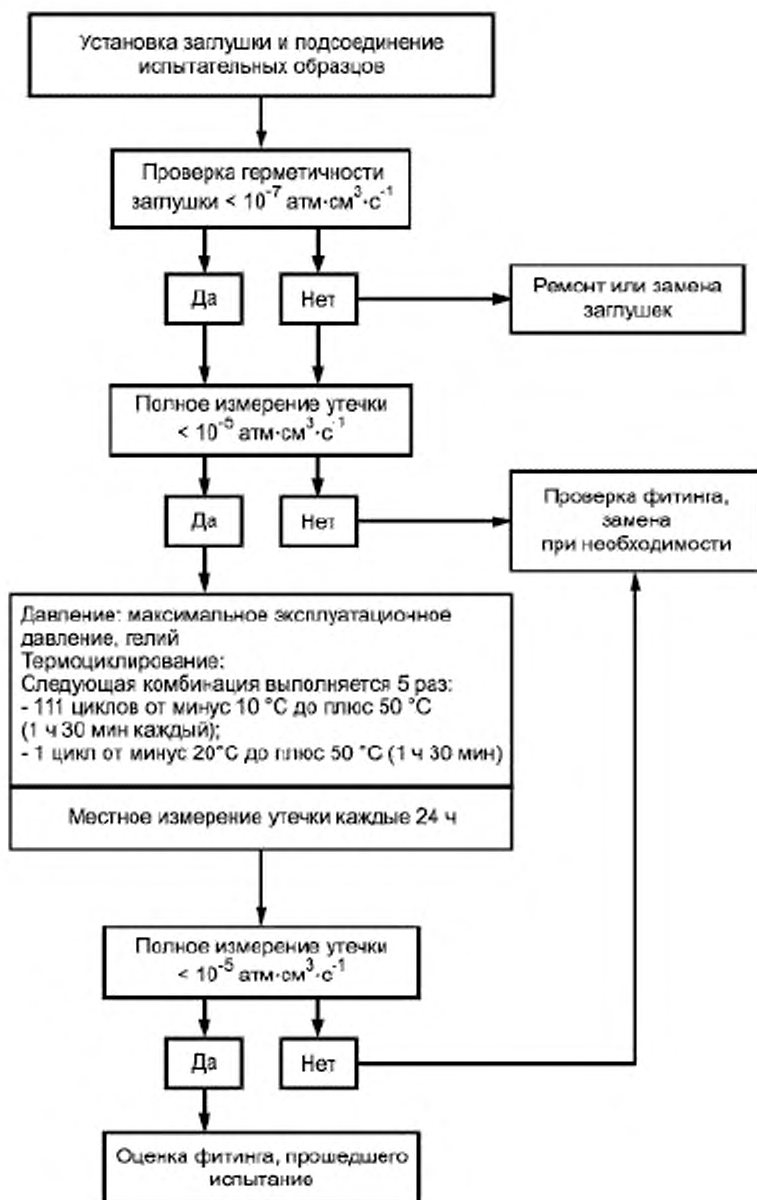
Рисунок И.2 – Испытание фитинга на герметичность
