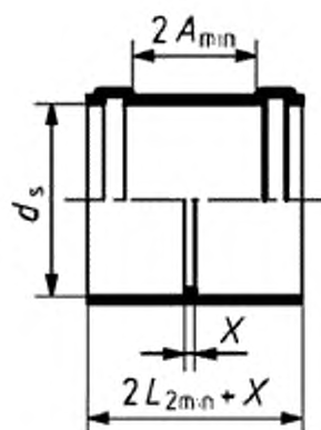
Рисунок 7 – Муфта
