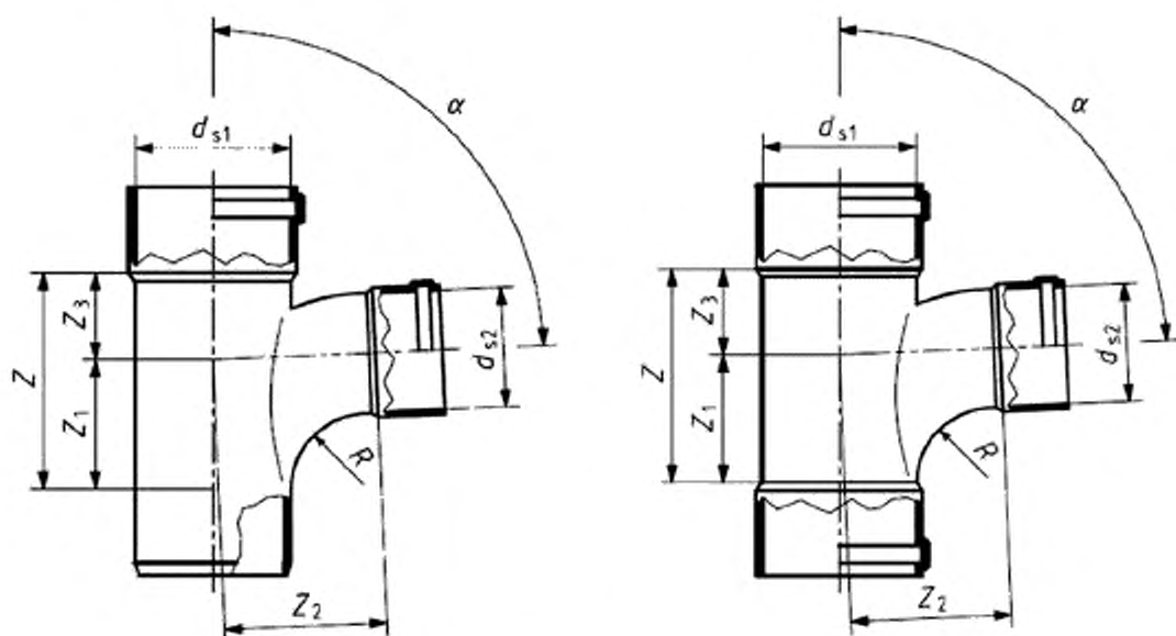
Рисунок 9 – Тройник
