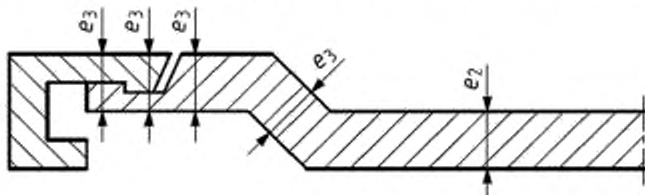
Рисунок 5 – Толщина стенки раструба с крышкой для установки уплотнительного кольца
