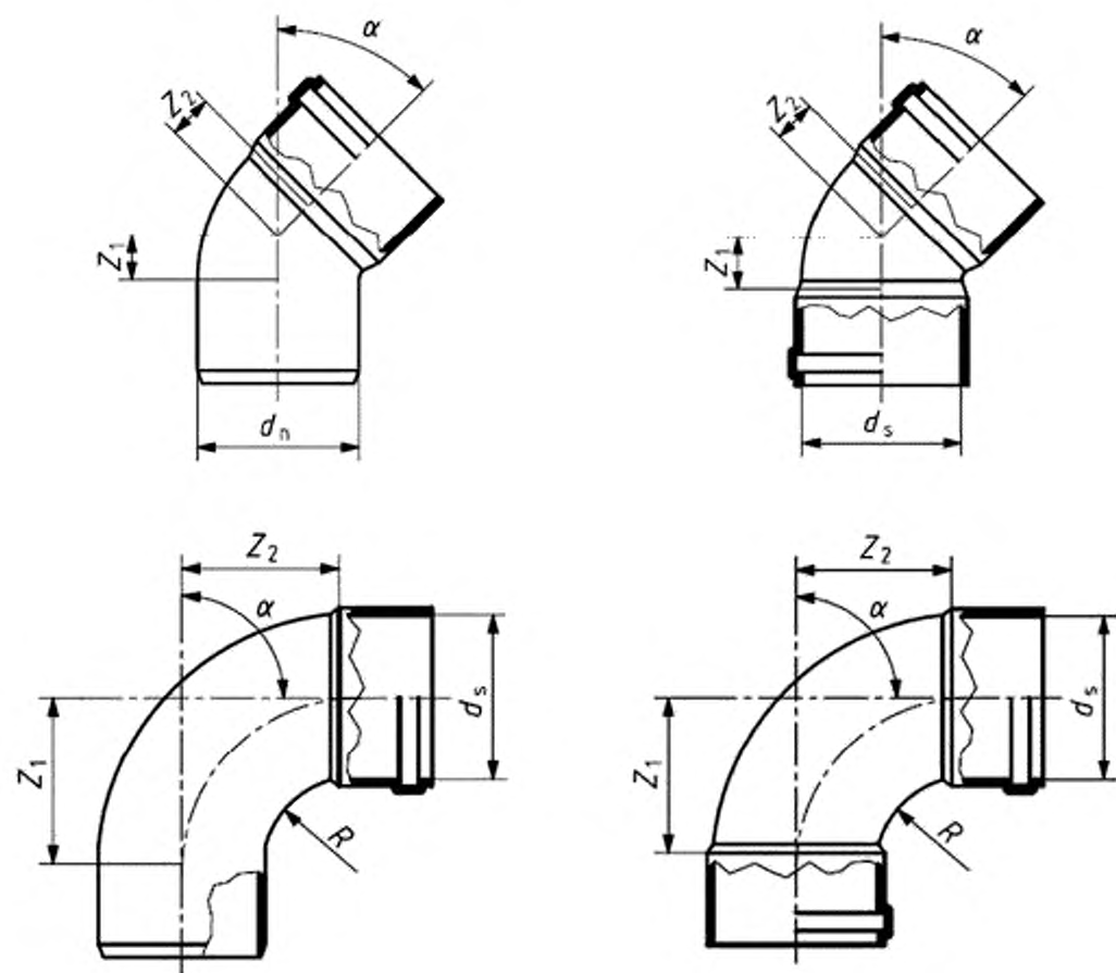
Рисунок 6 – Отвод
