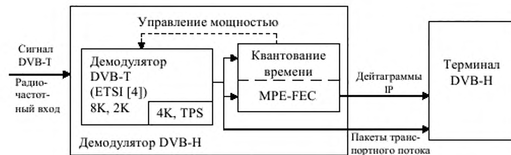
Рисунок 1 – Концептуальная структура приемника DVB-H
