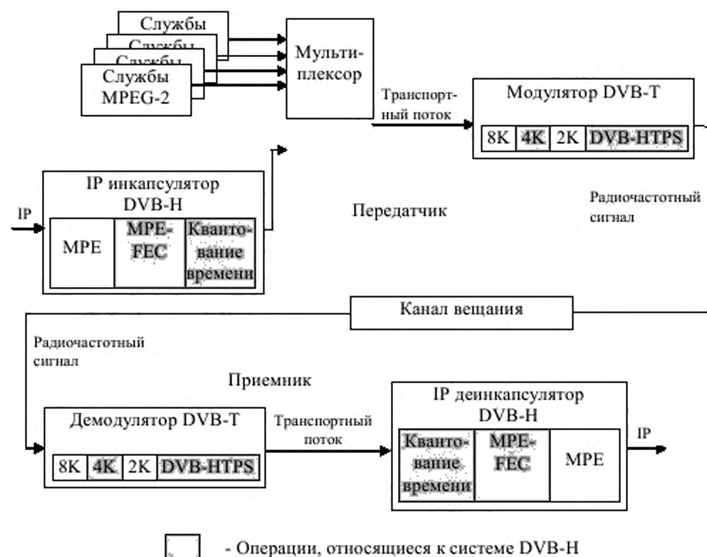
Рисунок 2 – Концептуальная структура системы DVB-H
