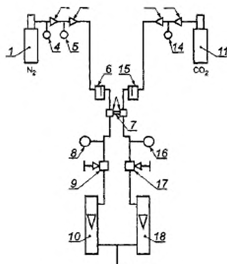
1 — баллон с азотом (аргоном); 2,12 — редукторы высокого давления; 3, 13 — редукторы низкого давления; 4, 5, 14 — манометры; 6, 15 — фильтры; 7 — переключатель потоков; 8, 16 — манометры 2,5 атм; 9, 17 — регуляторы расхода газа; 10, 18 — ротаметры; 11 — баллон с углекислым газом
