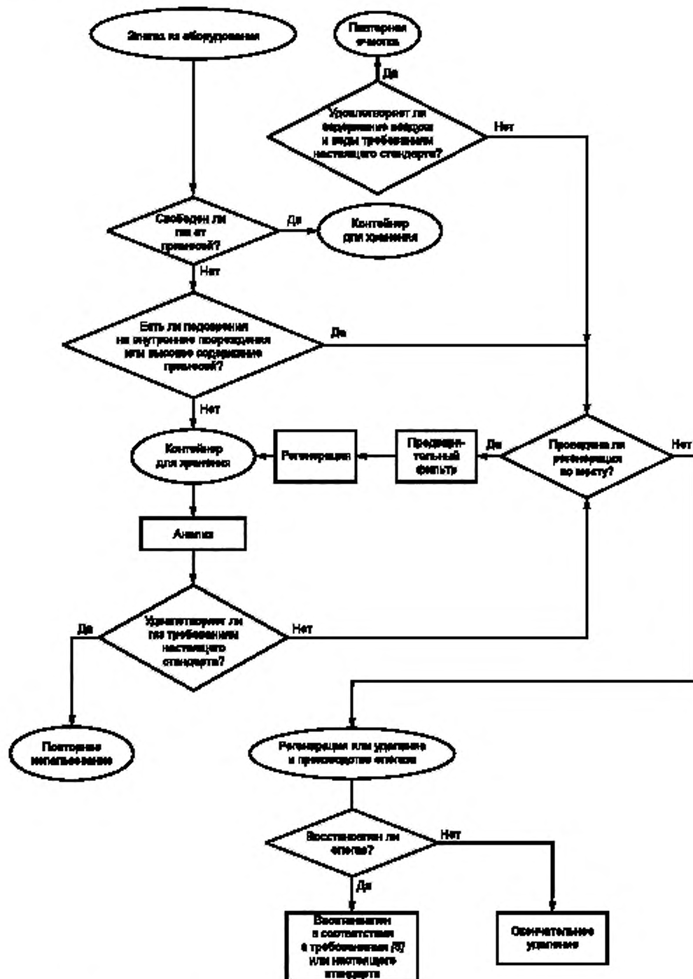
Рисунок 1 — Блок-схема для принятия решений по размещению или удалению аэгаза
