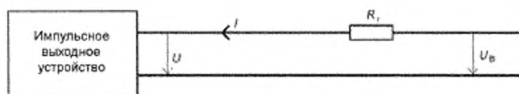
Рисунок С.1 – Испытательная схема импульсного выходного устройства
