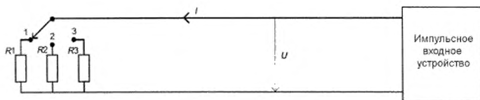
Рисунок D.1 – Испытательная схема импульсного входного устройства
