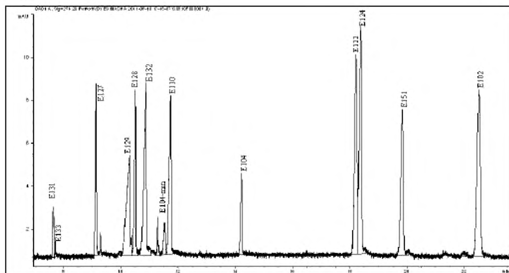
Рисунок 1 – Пример электрофореграммы смеси пищевых красителей на длине волны 254 нм
