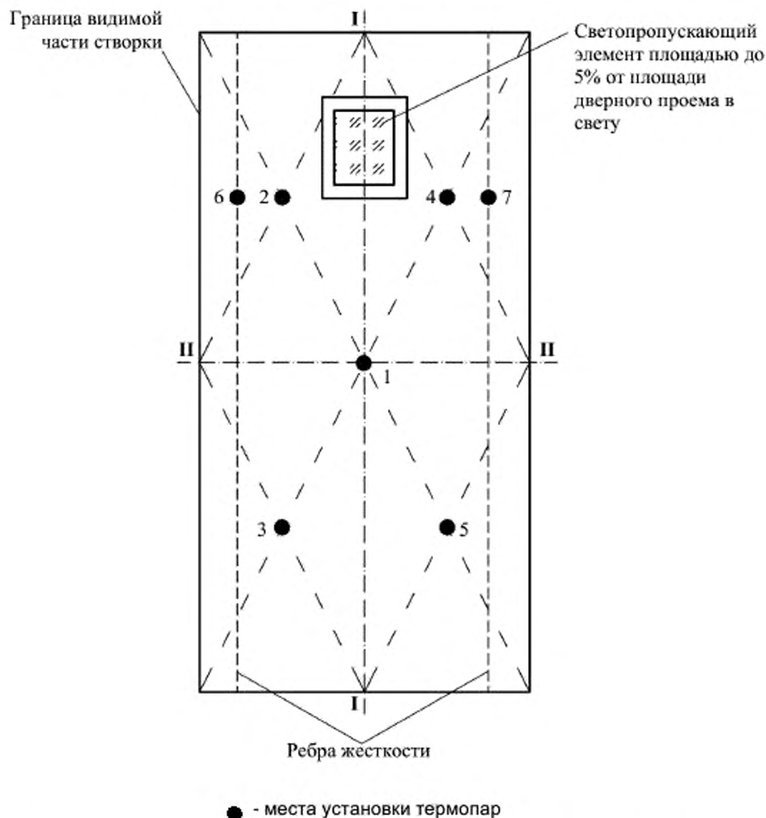
Рисунок А.1 - Схема установки термопар на необогреваемой поверхности створок одностворчатой распашной и сплошной горизонтально-раздвижной двери бокового открывания и со светопрускающим элементом створок до 5% от площади дверного проема в свету
