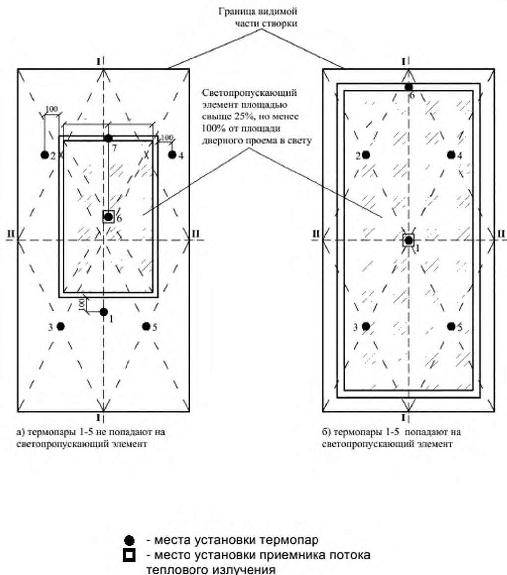
Рисунок А.3 - Схема установки термомпар и приемника потока теплового излучения на необогреваемой поверхности створки одностворчатой распашной и горизонтально-раздвижной двери бокового открывания со светопроницающим элементом створки свыше 25% но не менее 100% от площади проема в свету
