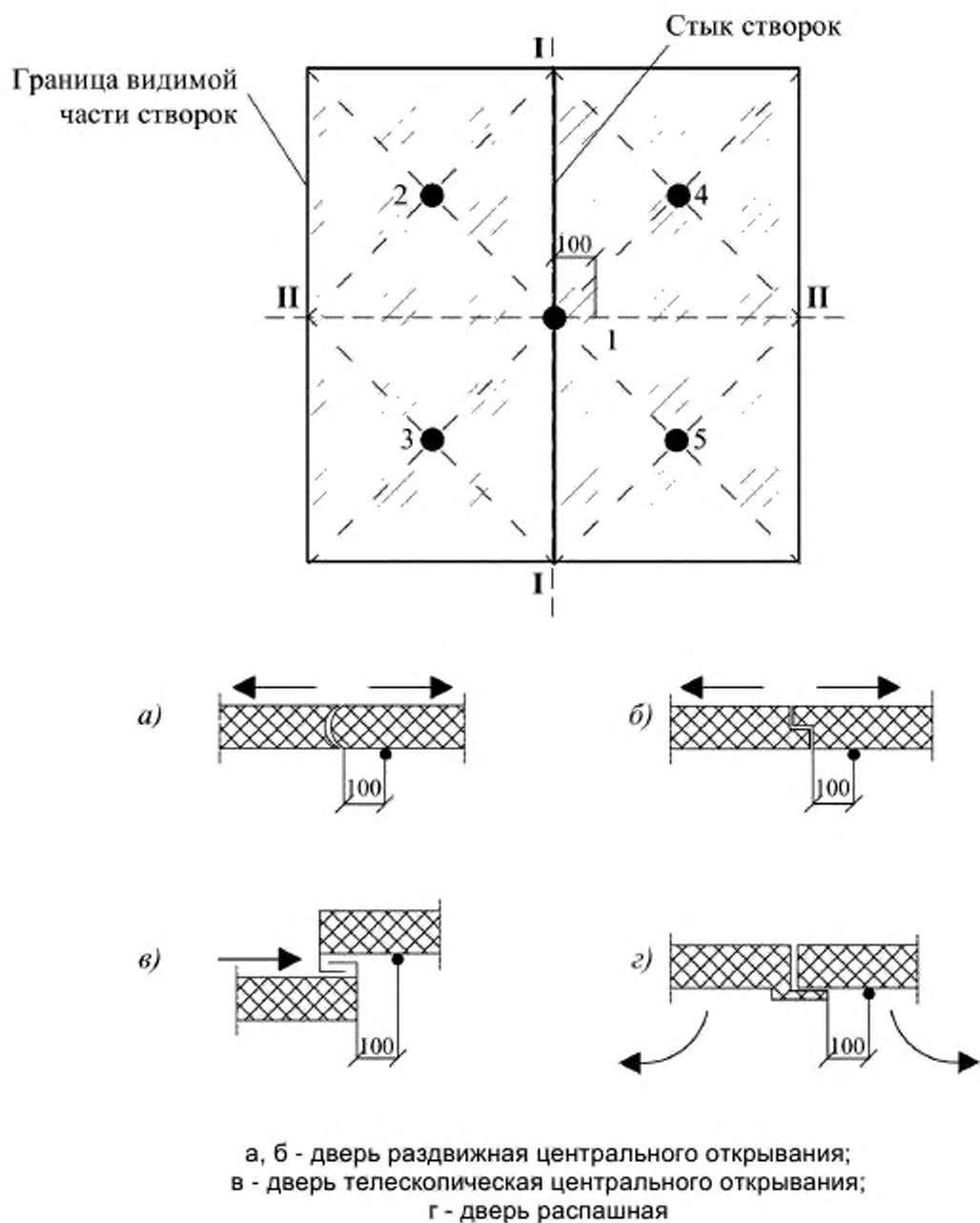
Рисунок А.4 - Схема установки термопар на необогреваемой поверхности двухстворчатой двери
