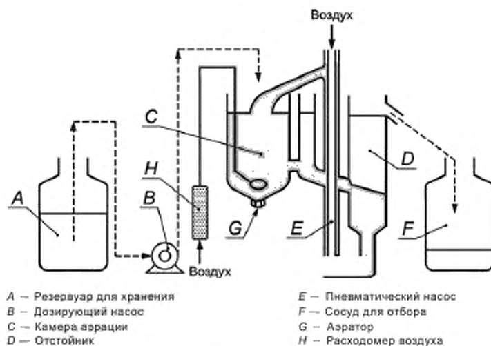
Рисунок 1 — Оборудование, применяемое для оценки биоразложения
