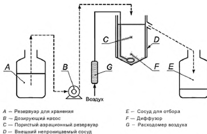
Рисунок 2 — Оборудование, применяемое для оценки биоразложения
