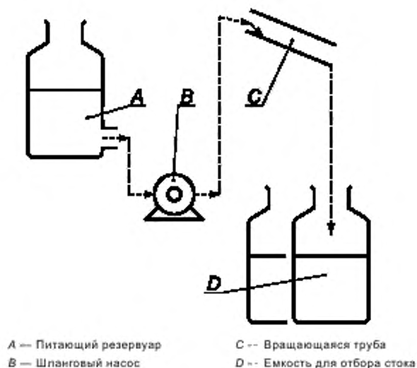
Рисунок 4 — Технологическая схема
