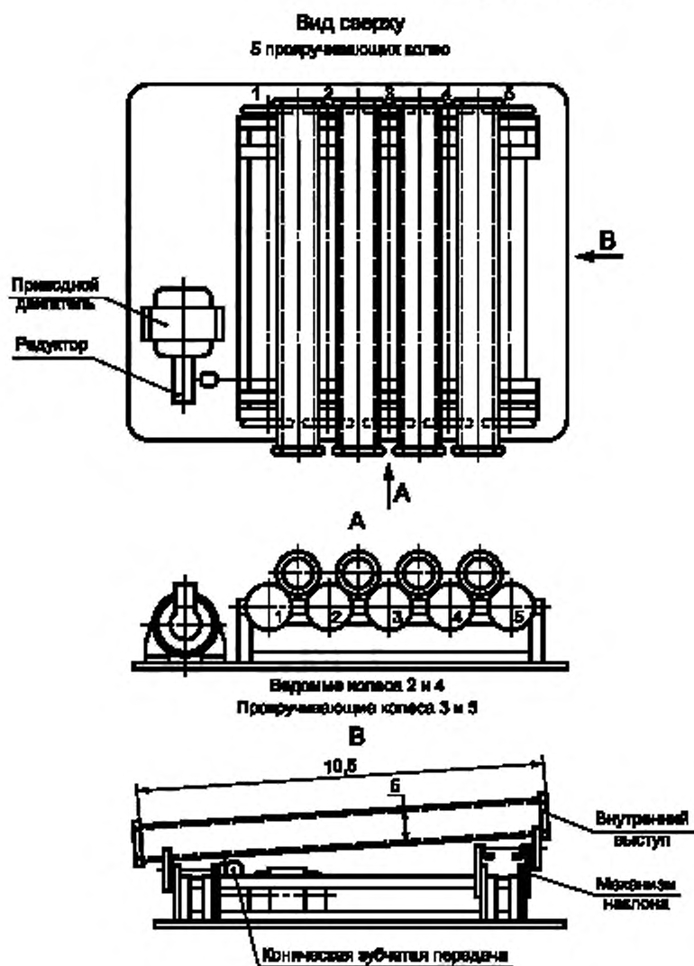
Рисунок 3 — Вращающиеся трубы
