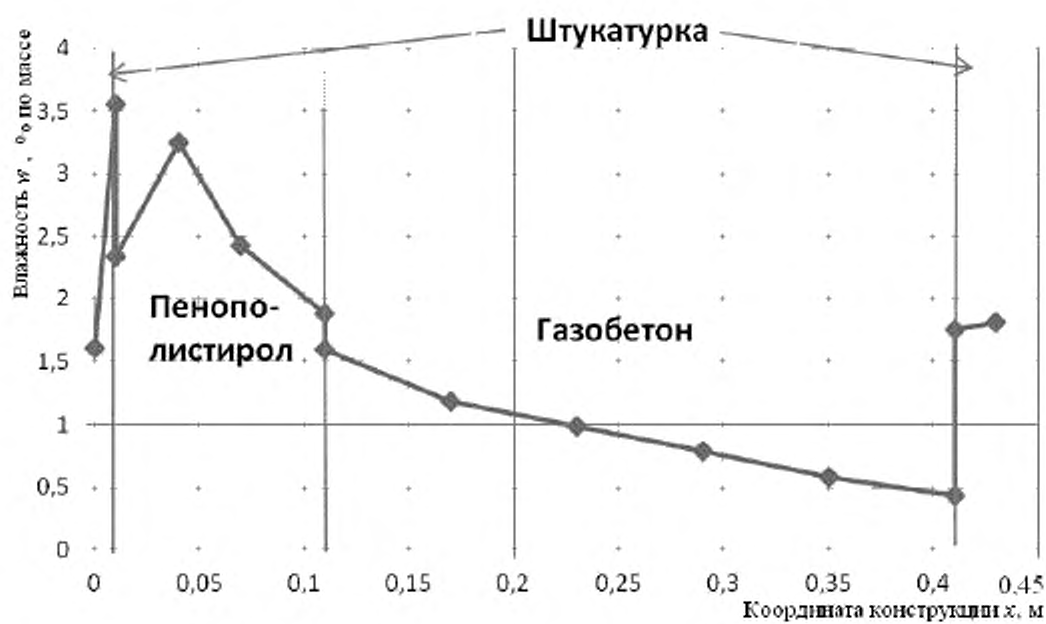
Рисунок Г.1 – Распределение влажности внутри конструкции
