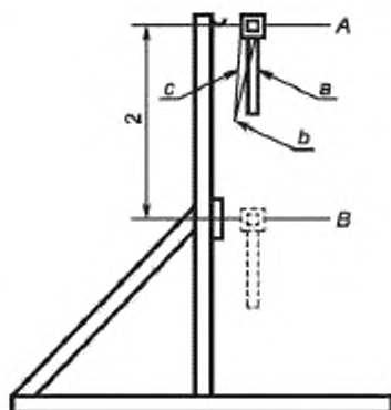
Рисунок А.1 — Испытание на механический удар
