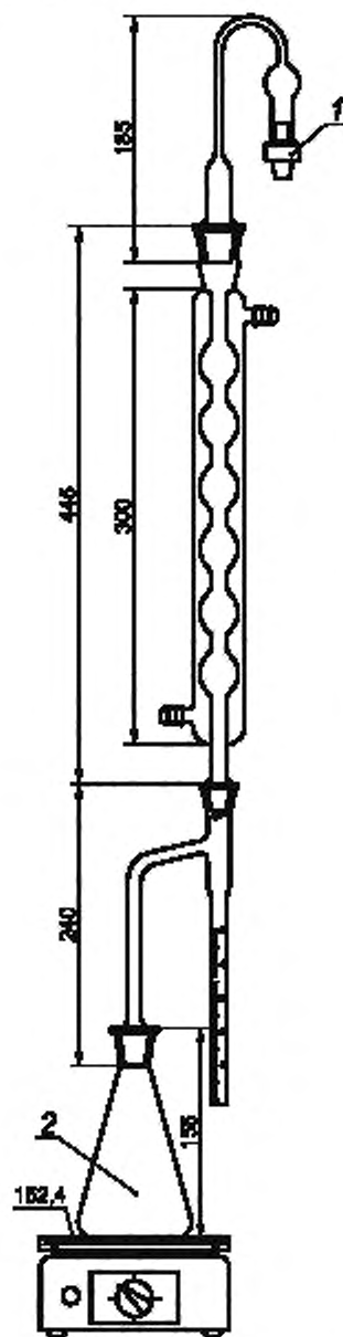
Рисунок 1 — Аппарат для определения содержания влаги
