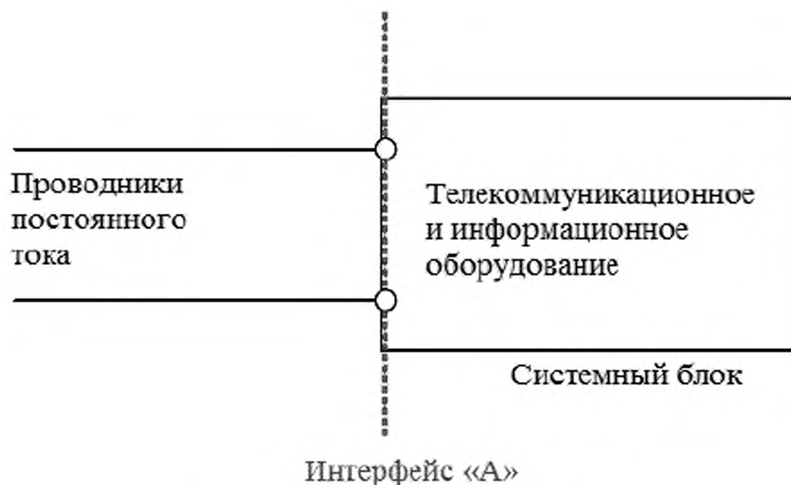
Рисунок 1 - Идентификация интерфейса «А»
