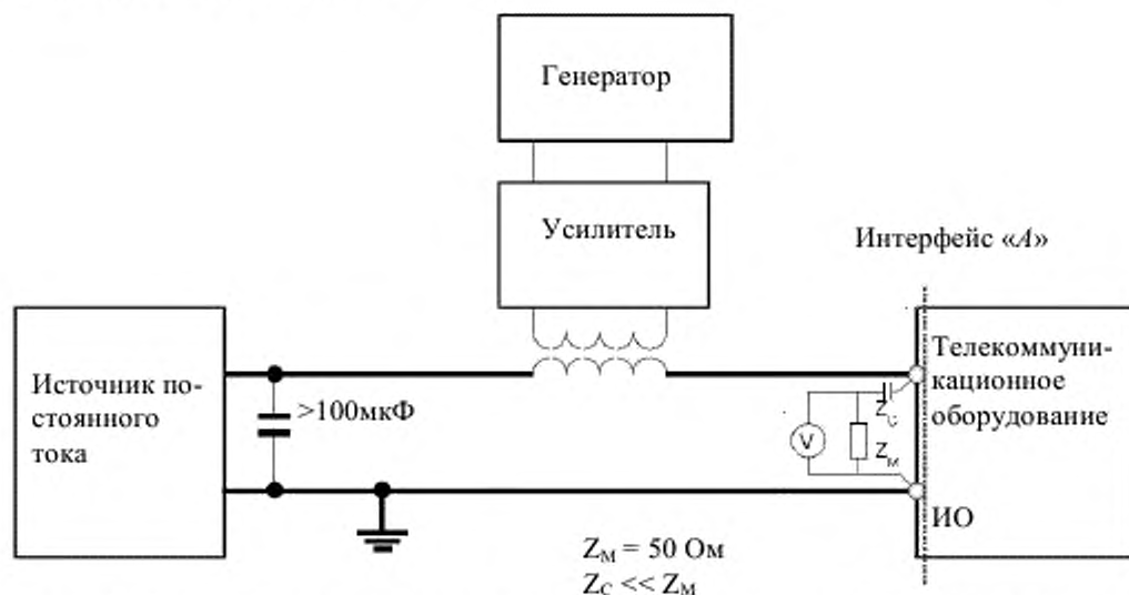
Рисунок 5 - Пример типовой испытательной схемы для испытания устойчивости к узкополосному шуму на интерфейсе «А»
