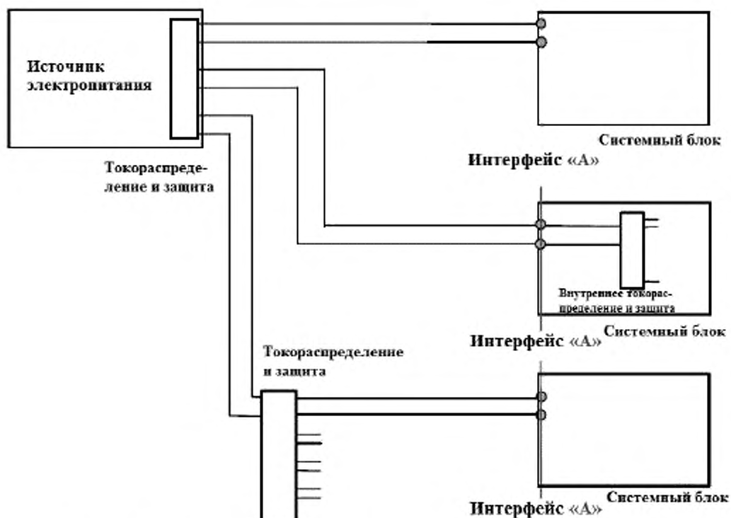
Рисунок А.1 - Идентификация интерфейса «А» (три предложенных примера)
