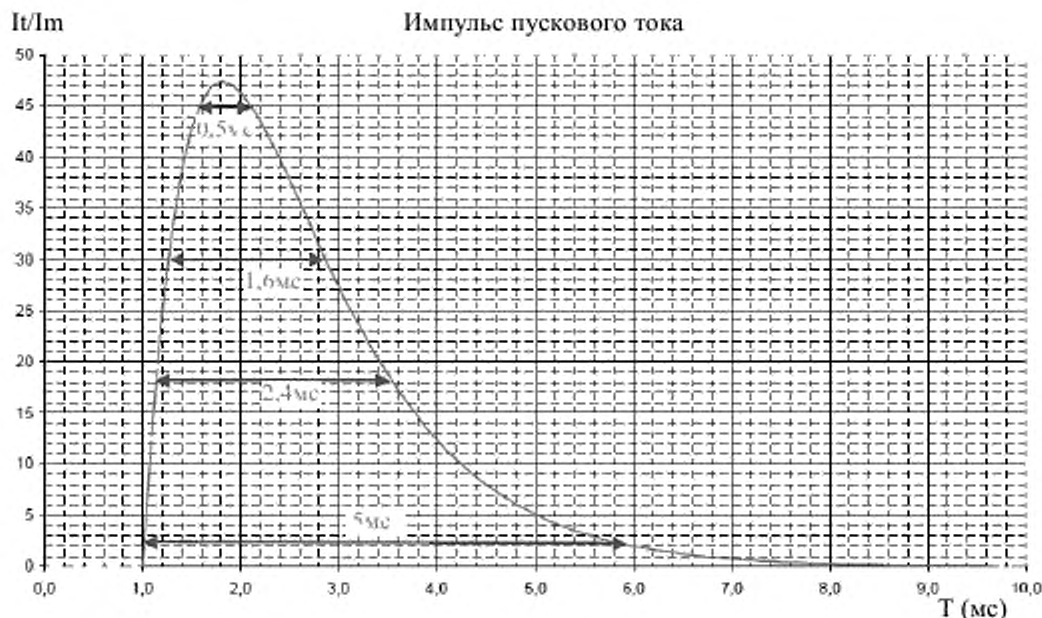
Рисунок В.1 - Пример импульса тока и связанных с ним измерений
