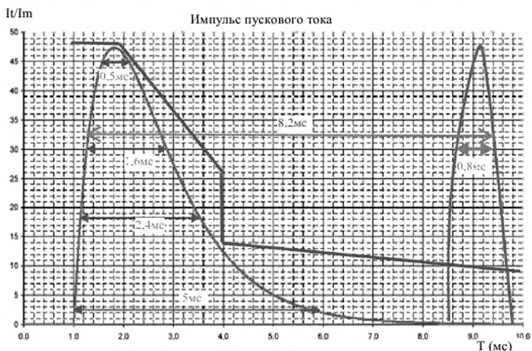
Рисунок В.3 - Полученная ширина достигается сложением ширины отдельных импульсов (1,6 мс + 0,8 мс)
