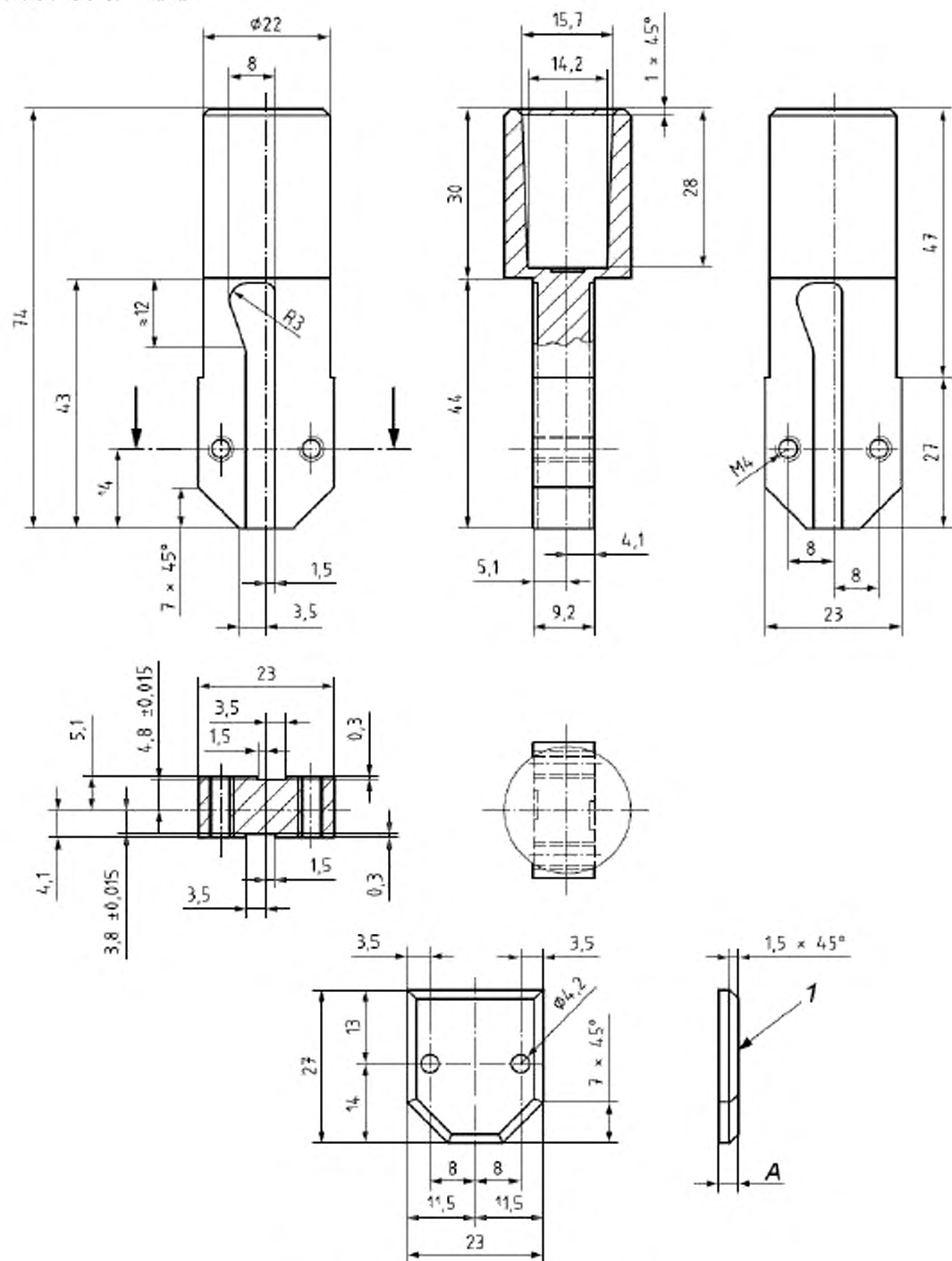
Рисунок А.1 — Специальный инструмент-держатель сменных ножей
