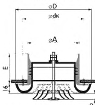
Рисунок 1 – Конструктивная схема диффузора веерного
