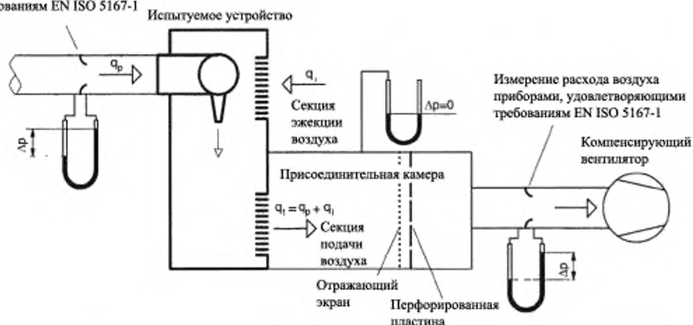
Рисунок 3 - Испытательная установка для измерения коэффициента эжекции методом нулевой разности давлений
