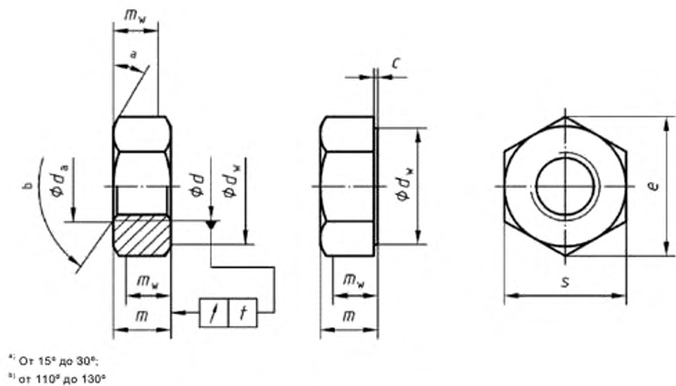
Рисунок 3 — Размеры гаек
