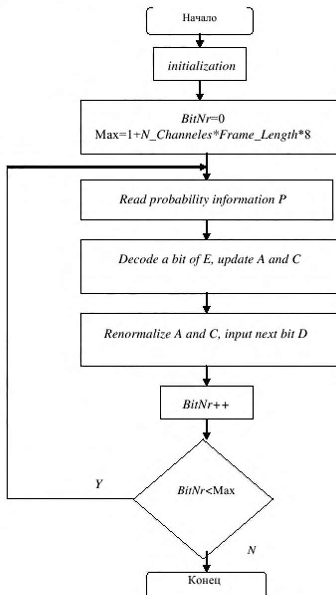
Рисунок 2 – Блок-схема арифметического декодера
