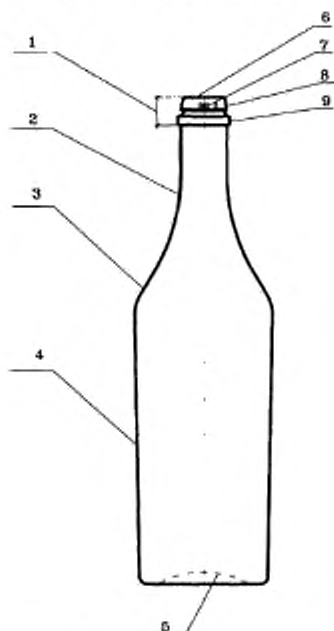
Рисунок А.1 – Конструкция бутылки
