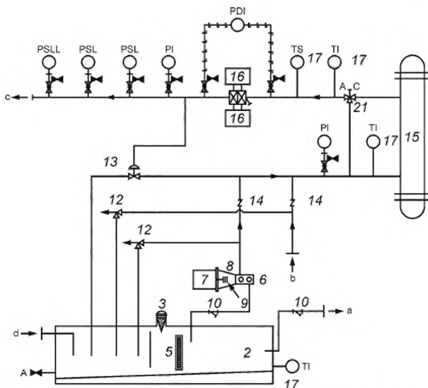
Рисунок Б.8 — Класс II-P0-R1-H0-BP0-C1F2-C0-PV1-TV1-BB0 или Класс II-P0-R1-H0-BP1-C1F2-C0-PV1-TV1-BB0
