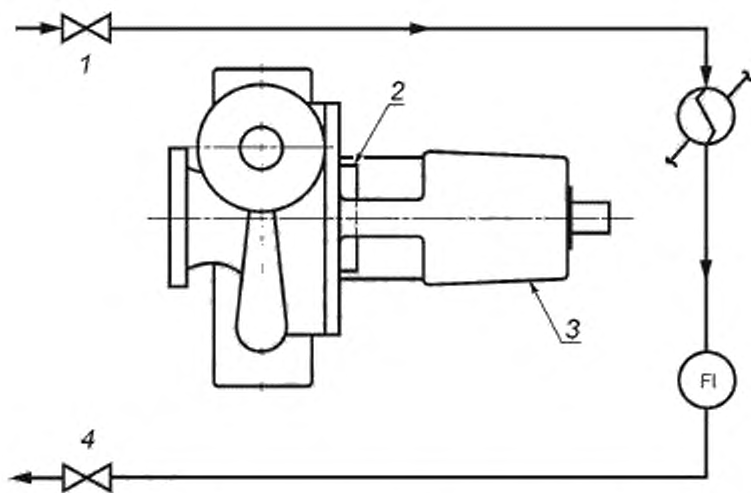
1 — впускной клапан; 2 — уплотнение; 3 — корпус подшипника; 4 — выпускной клапан
