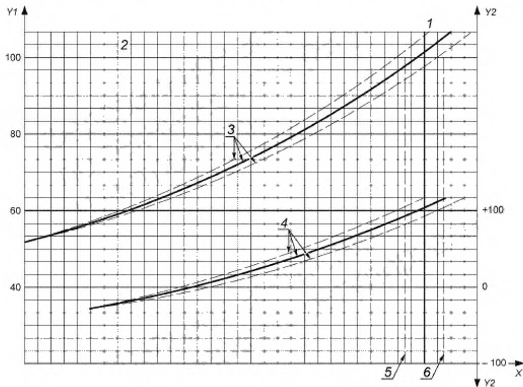
Рисунок В.2 — Испытательные допуски на параметры HPRT
