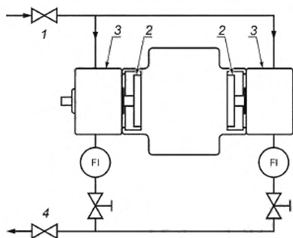
1 — впускной клапан; 2 — уплотнение; 3 — корпус подшипника; 4 — выпускной клапан
