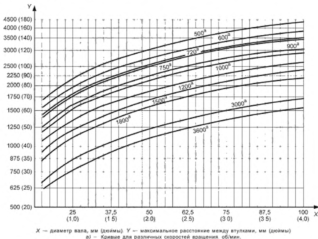
Рисунок 37 — Максимальное расстояние между направляющими втулками вала
