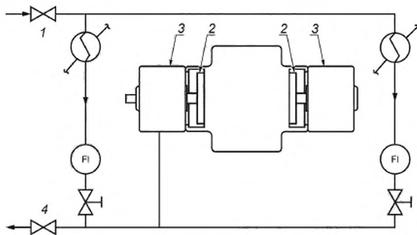
1 — впускной клапан; 2 — уплотнение; 3 — корпус подшипника; 4 — выпускной клапан
