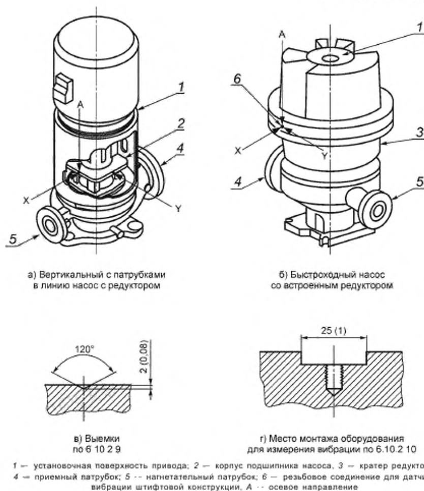
Рисунок 33 — Положения для снятия показаний вибрации: а — на вертикальном линейном и б — на быстроходном насосе со встроенным редуктором
