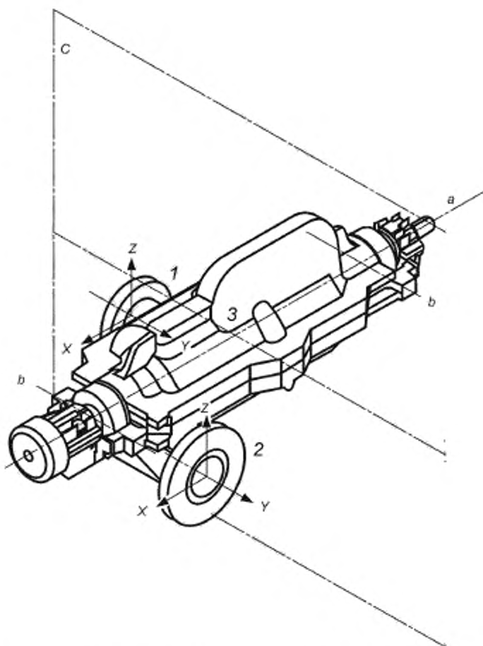
1 — выходной патрубок; 2 — входной патрубок; 3 — осевая линия насоса; а — ось вала; б — ось опорной плиты; с — вертикальная плоскость
