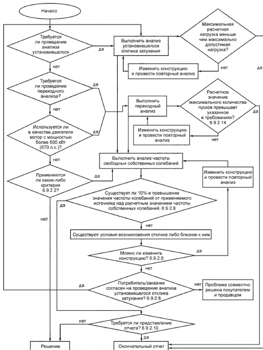
Рисунок 29 — Алгоритм анализа крутильных колебаний
