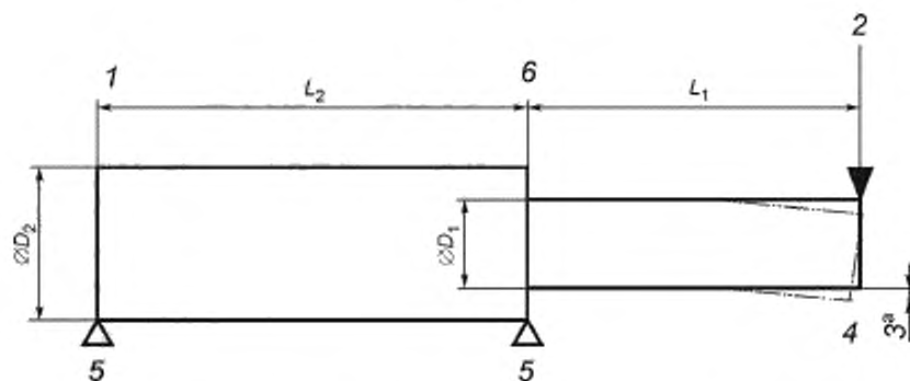
1 — упрощенный вал; 2 — радиальная нагрузка на крыльчатку; 3 — отклонение; 4 — сторона рабочего колеса; 5 — опора (подшипник); 6 — консольный насос;
