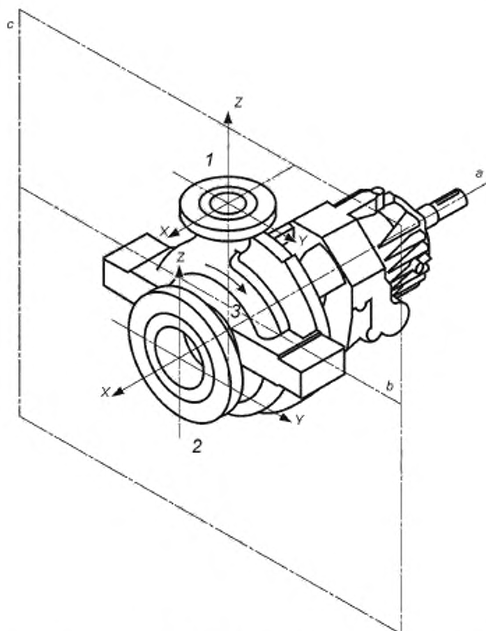
1 -- нагнетательный патрубок; 2 -- всасывающий патрубок; 3 -- центр насоса; а -- ось вала; б -- ось основания; с -- вертикальная плоскость
