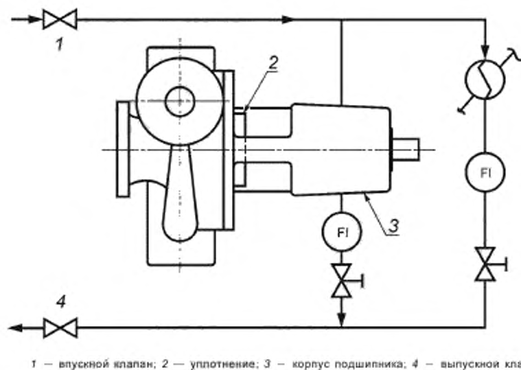
Рисунок Б.3 — Трубопровод для консольных насосов — Схема К, охлаждение корпуса подшипника параллельным потоком, идущим в теплообменник
