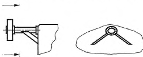
Рисунок 20 — Типовая конструкция ребер жесткости
