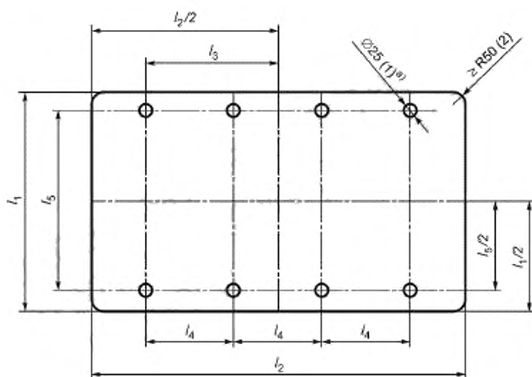
Рисунок Г.1 — Стандартная опорная плита
