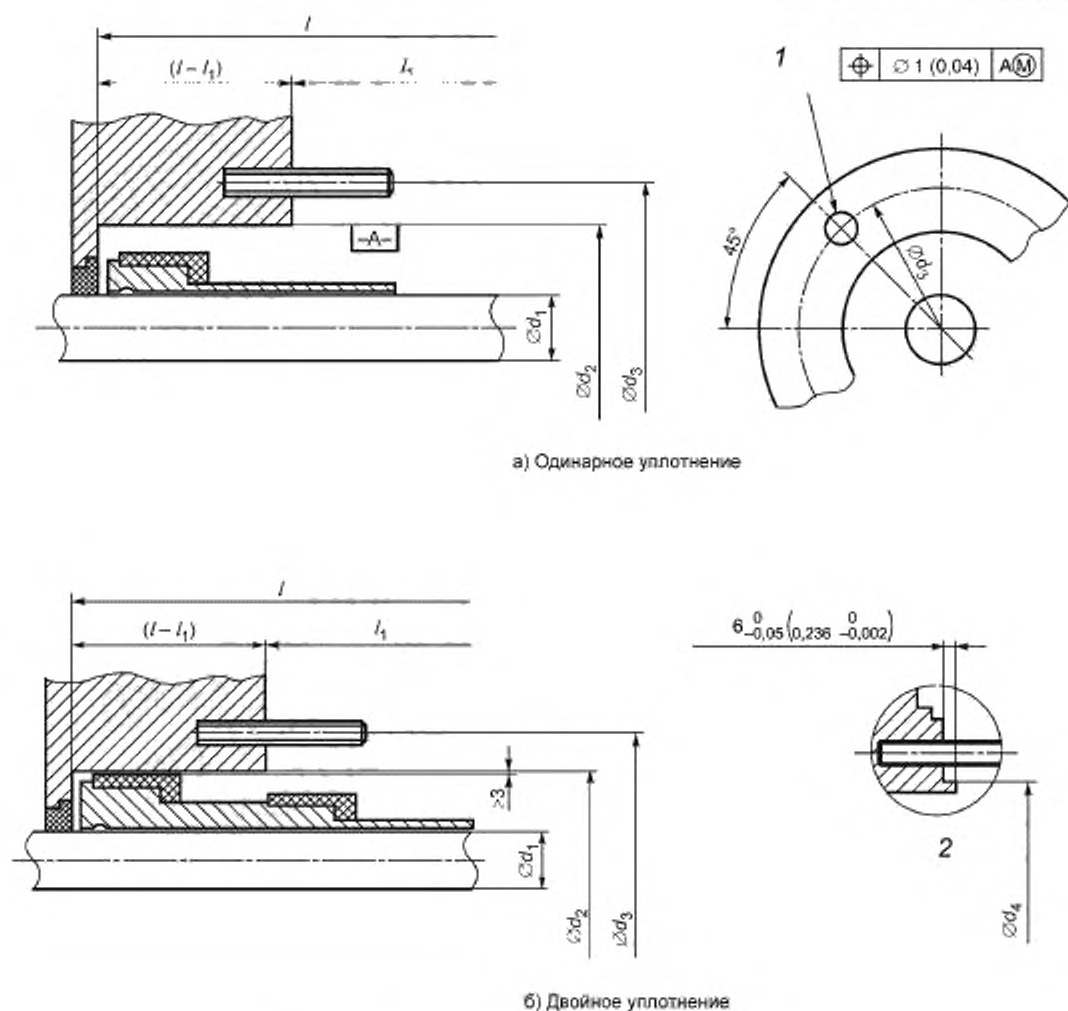
б) Двойное уплотнение
