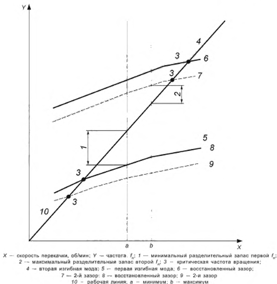
Рисунок К.2 — Типичная диаграмма Кэмпбелла
