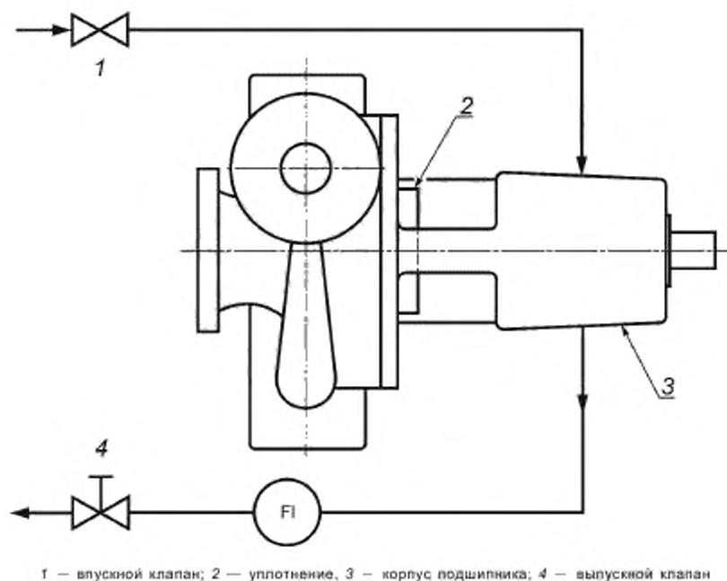
Рисунок Б.2 — Трубопровод для консольных насосов — Схема А, охлаждение корпуса подшипника
