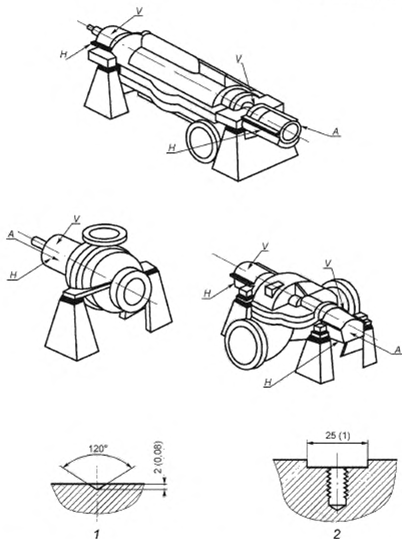
Рисунок 31 — Места измерения вибрации на горизонтальных насосах
