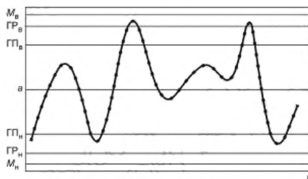
Рисунок Г.2 — Контрольная карта скользящих средних
