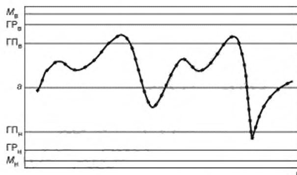
Рисунок Г.2 — Контрольная карта скользящих средних
