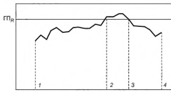
Рисунок Г.4 — Контрольная карта размахов
