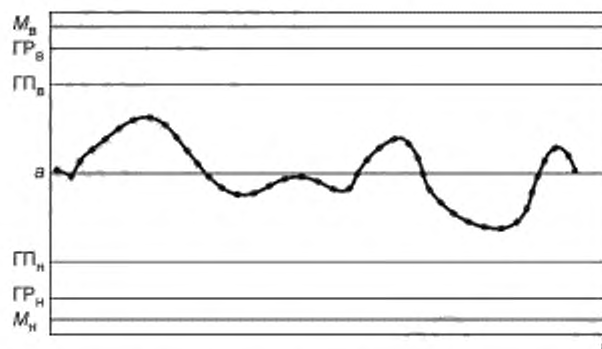
Рисунок Г.1 — Контрольная карта скользящих средних
