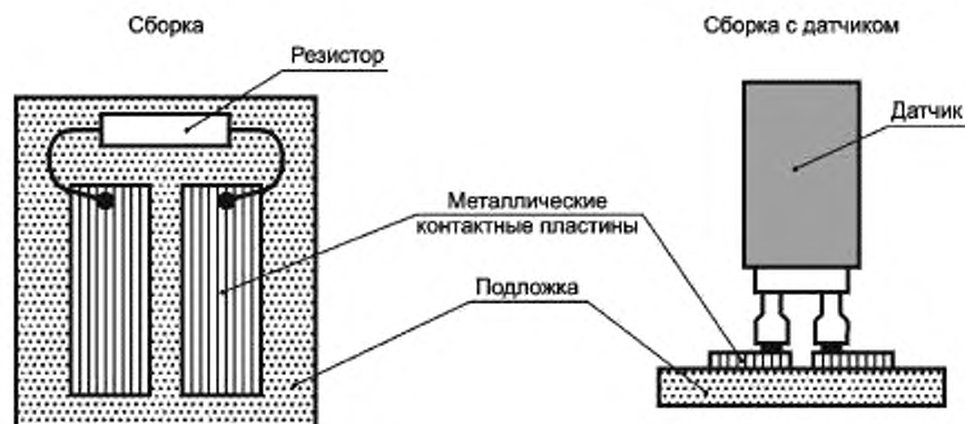
Рисунок 3 — Сборка для проверки сопротивления
