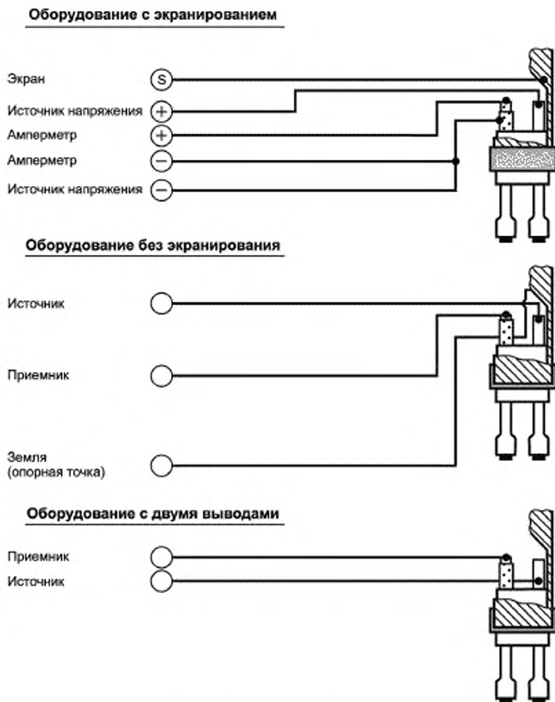
Рисунок 2 — Соединение датчика с измерительным оборудованием
