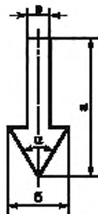
B = 180-200 мм; b = 60-100 мм; H = 30-40 мм; \alpha = 60^\circ-70^\circ
