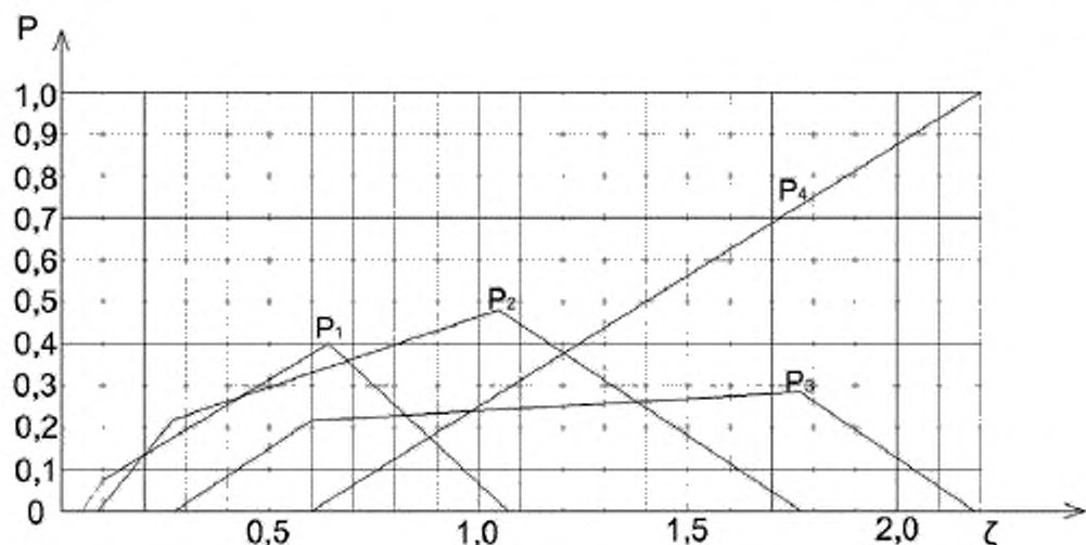
Рисунок 4.1 - Вероятности различной степени разрушения здания (сооружения) и повреждения технологического оборудования в зависимости от величины обобщенного показателя устойчивости, \xi_o(\xi_{ro})
