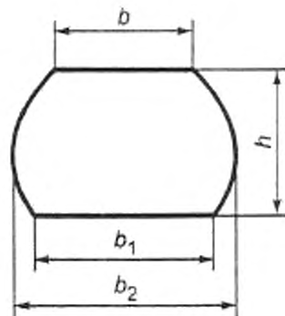
Рисунок 2 – Поперечное сечение бруса вида Б
