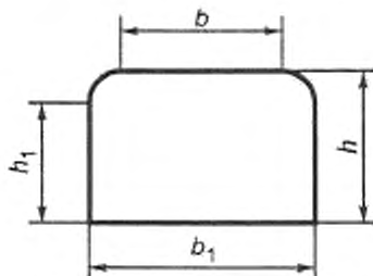
Рисунок 1 – Поперечное сечение бруса вида А
