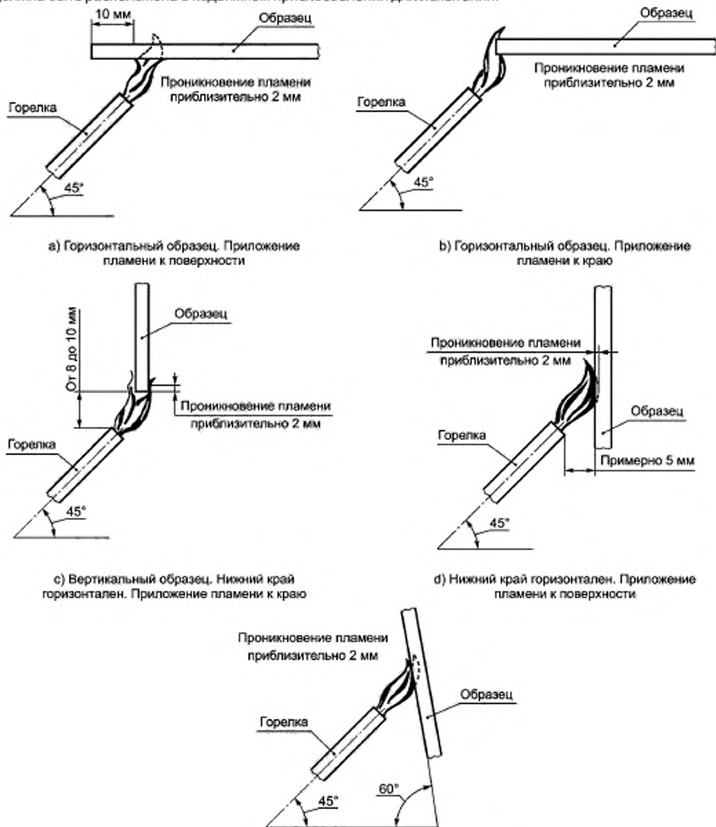
е) Испытание с использованием горелки игольчатого типа. Виды сбоку на тест-плату и горелку
