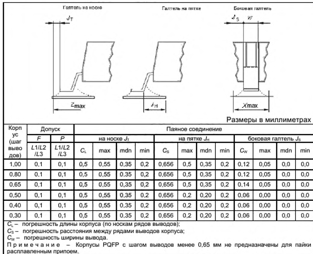
Рисунок 3 – Анализ формы паяного соединения
