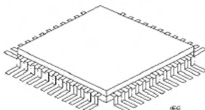
Рисунок 9 – корпус типа PLQFP (квадратный)
