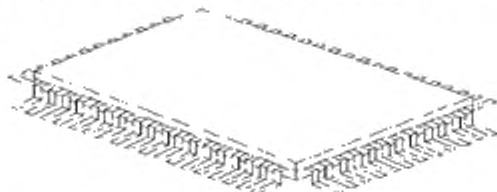
Рисунок 13 – Конструкция корпуса типа PLQFP (прямоугольный)
