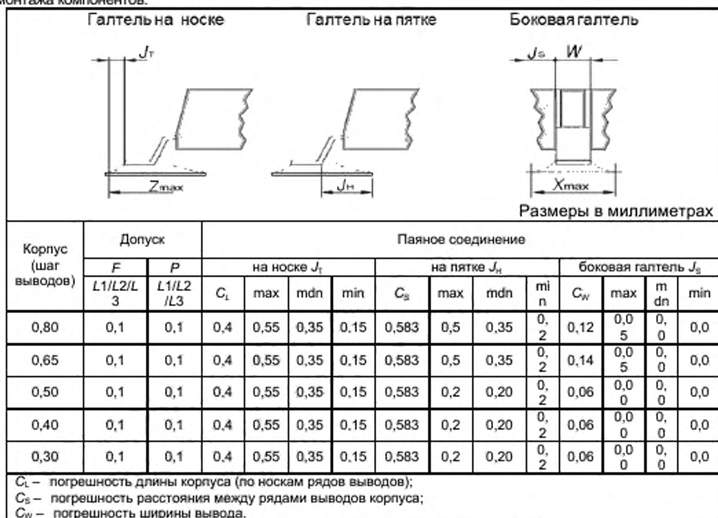
Рисунок 19 – Анализ формы паяного соединения
