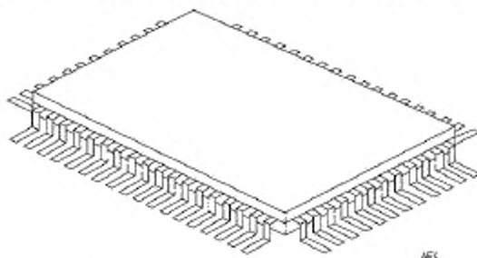
Рисунок 5 – Конструкция корпуса типа PQFP (прямоугольный)
