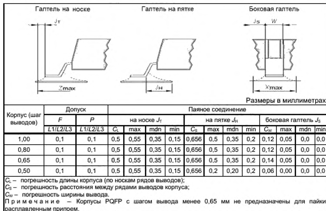
Рисунок 7 – Анализ формы паяного соединения
