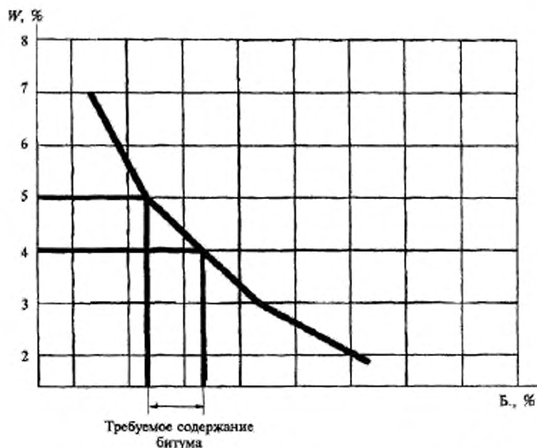
Рисунок 2 – Определение требуемого содержания битума
