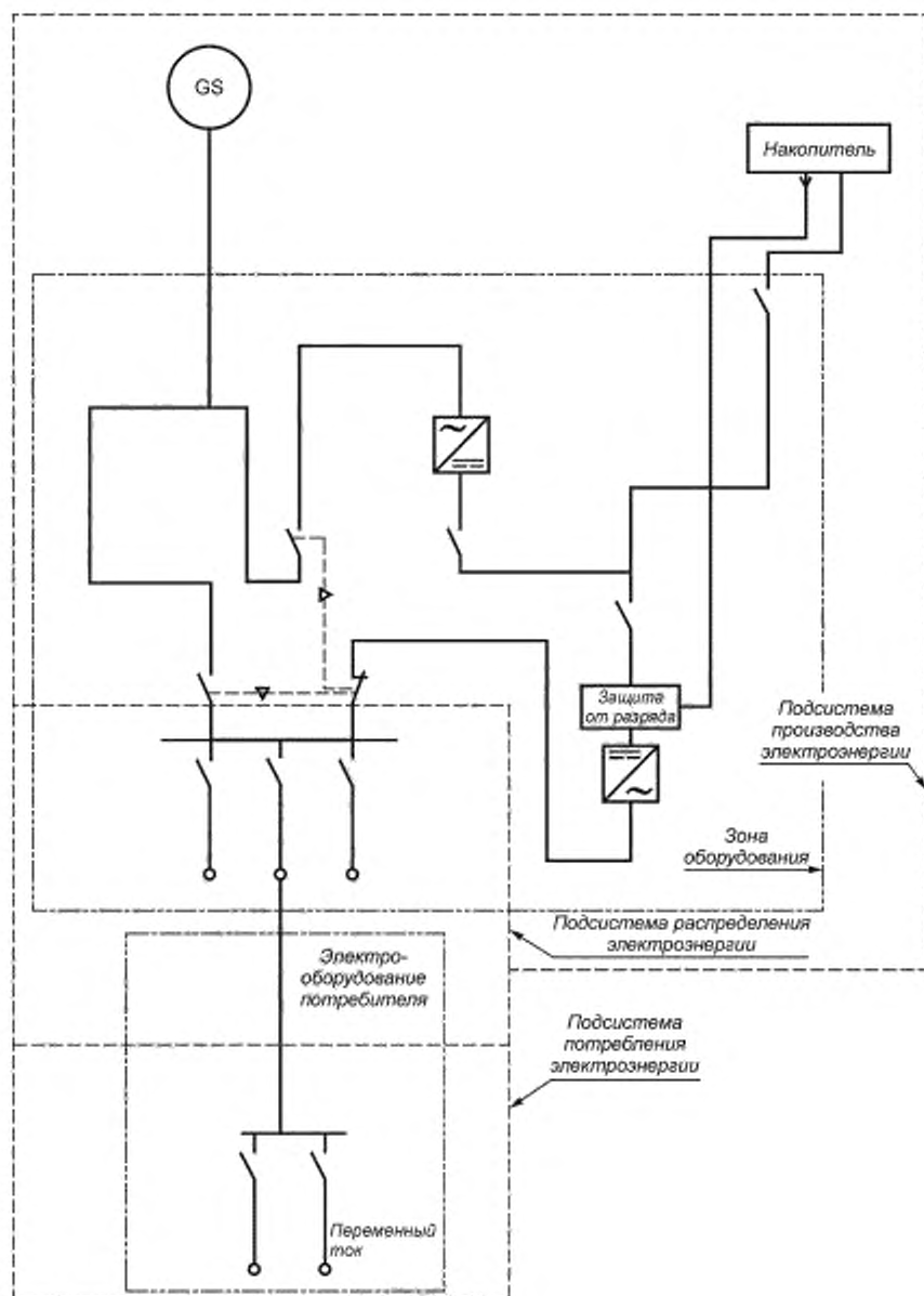
Рисунок Д.18 — Система типа Т 6 С
