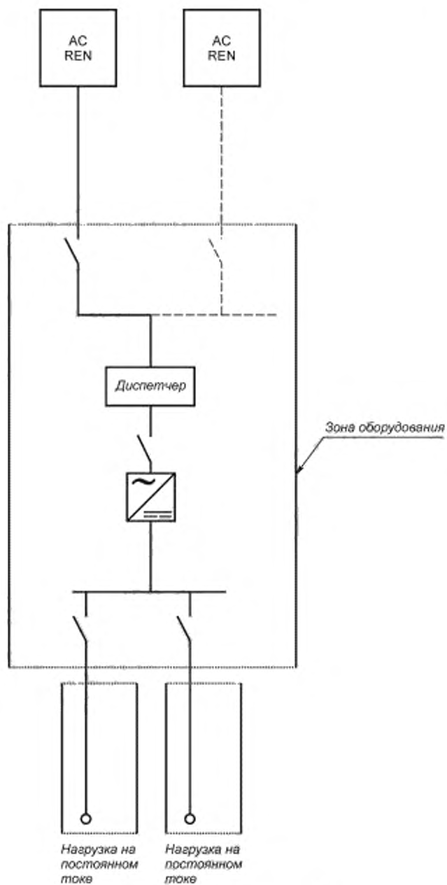
Рисунок Д.3 — Система типа Т 1 -с
