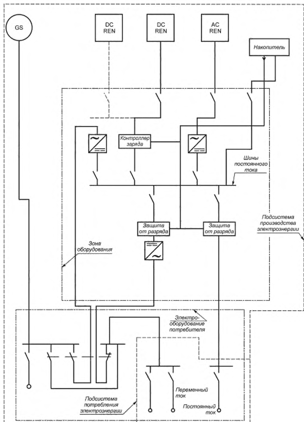
Рисунок Д.8 — Система типа T 4 1
