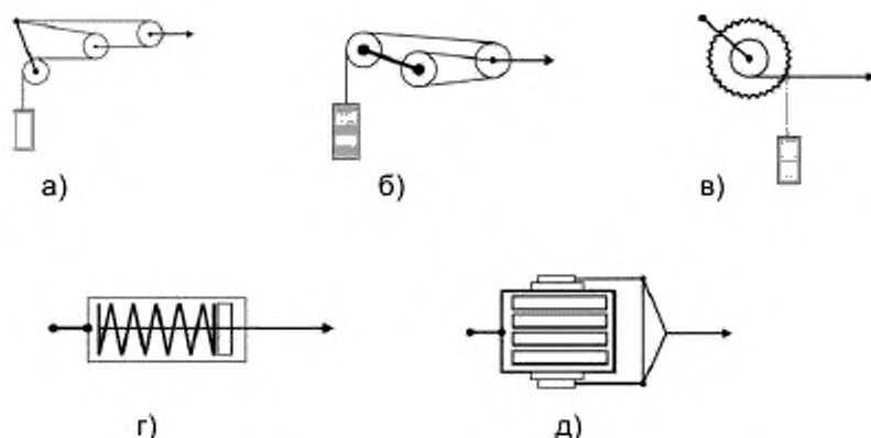
Рисунок 1 – Схематическое изображение компенсаторов
