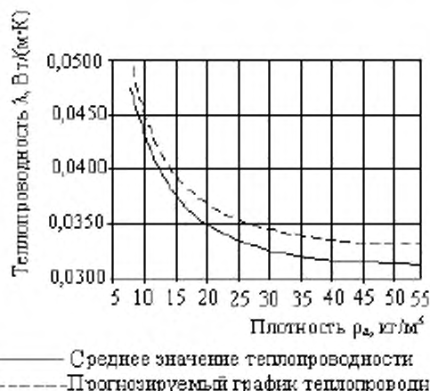
Рисунок В.2 – Зависимость теплопроводности от плотности (косвенный метод) [толщина материала 50 мм; средняя температура 10 °С; (1 - a) = 0,90 ; n = 3873 ]
