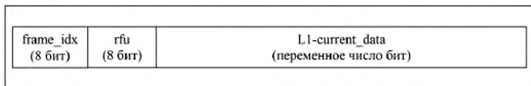
Рисунок 6 — Текущие L1-данные как полезная нагрузка
