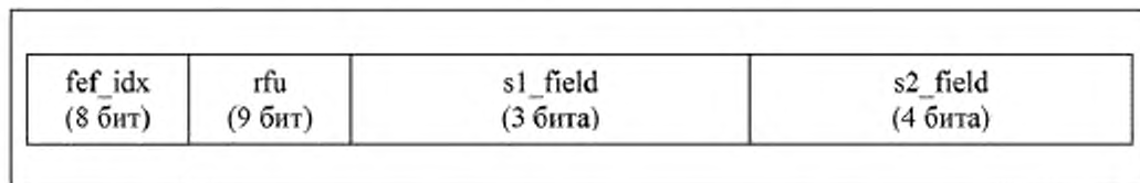
Рисунок 11 — Нулевой блок FEF как полезная нагрузка
