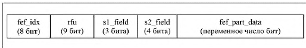
Рисунок 12 — Блок FEF с I/Q-данными как полезная нагрузка
