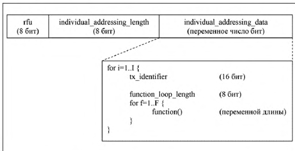
Рисунок 10 — Индивидуальная адресация как полезная нагрузка
