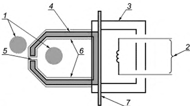
Рисунок D.1 — Части датчика тока (также см. таблицу D.101)
