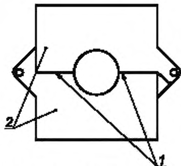
Тип С – Датчик тока с наборным сердечником
