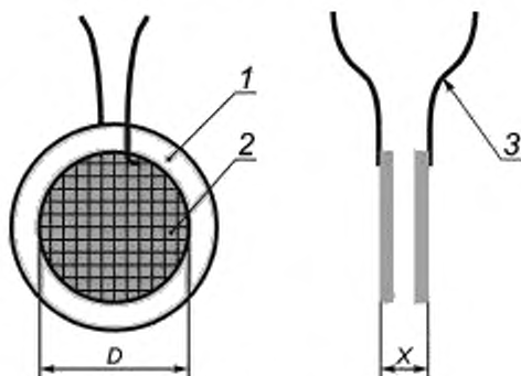
1 — непроводящий основной материал; 2 — проводящий поверхностный материал; 3 — испытательные токопроводящие проводники; D — диаметр проводящего поверхностного материала; X — предельная толщина испытательного щупа
