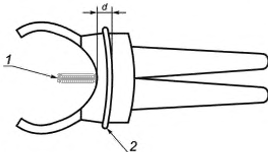
Рисунок 103 — ЗАЗОР между ЗАЩИТНЫМ БАРЬЕРОМ или тактильным индикатором и ЗАЖИМОМ и ОПАСНЫМ ДЛЯ ЖИЗНИ проводником
