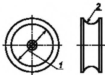
1 — внутренний диаметр шкива; 2 — радиус кривизны шкива
