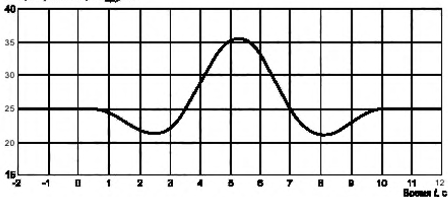
Рисунок 4 — Пример экстремального рабочего порыва ( N = 1 , V_{hub} = 25 м/с)
