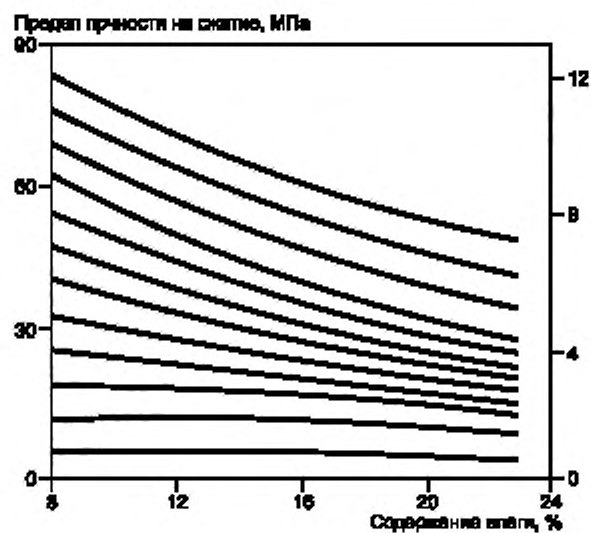
Рисунок Д.8 — Зависимость предельной прочности (при сжатии до образования щелок) древесины от влажности
