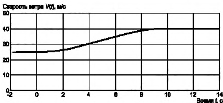
Рисунок 7 — Пример ЭКГ ветра ( V_{hub} = 25 м/с)
