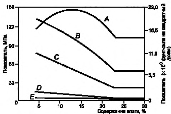
Рисунок Д.8 — Зависимость предельной прочности (при сжатии до образования щелок) древесины от влажности
