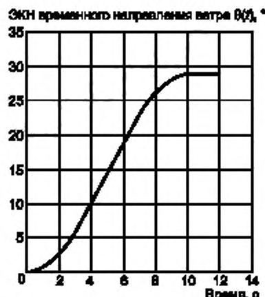
Рисунок 9 — Пример переходного процесса изменения направления ветра ( V_{hub} = 25 \text{ м/с} )
