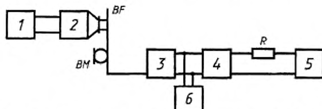
Рисунок Е.3 — Схема для испытания перенапряжением
