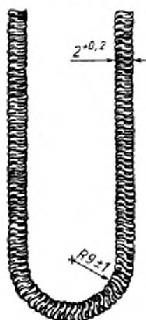
Рисунок Г.4 — Испытательная цепочка
