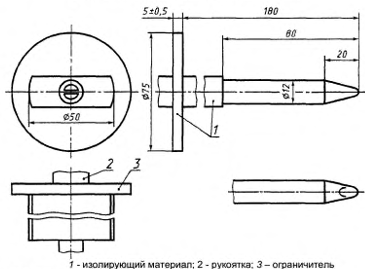
Рисунок Г.1 — Шарнирный испытательный палец
