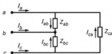
a, b, c — фазы основной вторичной обмотки ТН; I_a, I_b, I_c — фазные токи; I_{ab}, I_{bc}, I_{ca} — межфазные токи; Z_{ab}, Z_{bc}, Z_{ca} — межфазные нагрузки
