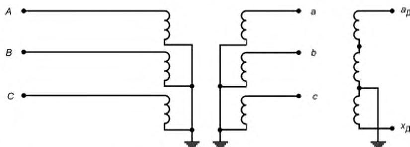
А, В, С — фазы первичной обмотки ТН; а, б, с — фазы основной вторичной обмотки ТН; а д , х д — фазы дополнительной вторичной обмотки ТН
