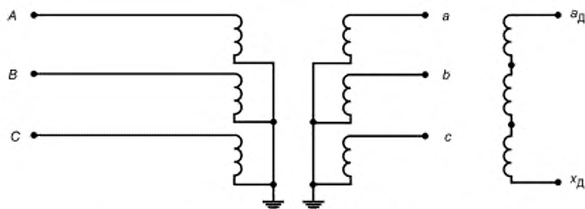
А, В, С — фазы первичной обмотки ТН; а, б, с — фазы основной вторичной обмотки ТН; а д , х д — фазы дополнительной вторичной обмотки ТН
