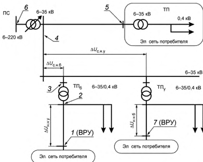
1, 7 — ВРУ; 2 — шины 0,4 кВ ТП, 3, 5 — шины 6—35 кВ ТП, 4 — шины 6—35 кВ ПС; 6 — шины 35—220 кВ ПС (ЦП)
