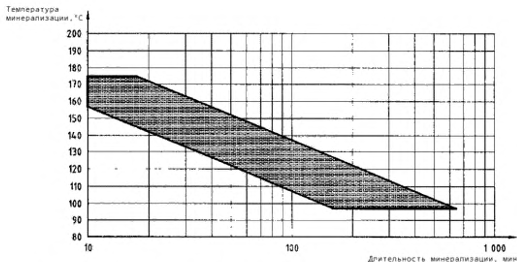
Рисунок 1 — Диапазон допускаемых значений температуры и длительности минерализации
