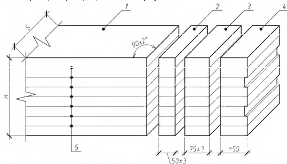
H и S — высота и ширина клеевого элемента; 1 — многослойный элемент; 2 — заготовка для выпилки образцов для предварительных испытаний на послойное скалывание; 3 — образец для испытаний на расслаивание; 4 — торцевой срез; 5 — клеевые швы
