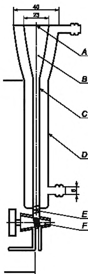
A — место соединения с муфтой из матового стекла; B — свободное пространство; C — внутренняя часть колонки; D — внешняя часть колонки; E — пробка из стекловолокна; F — залорный кран
