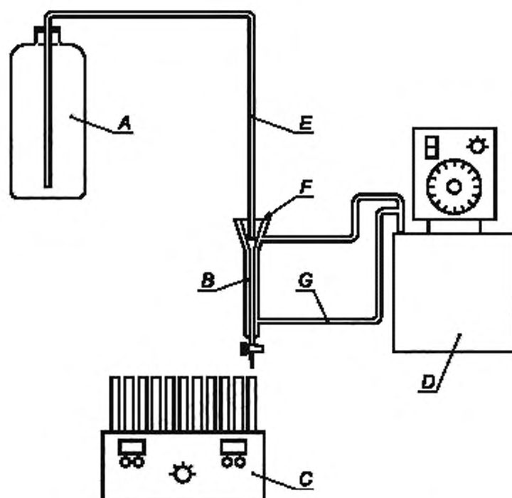
A — выравнивающий сосуд (например, 2,5 л колба); B — колонка; C — приемник фракций; D — термостат; E — тефлоновая трубка; F — соединение из матового стекла; G — трубка между термостатом и колонкой (внутренний диаметр 8 мм)
