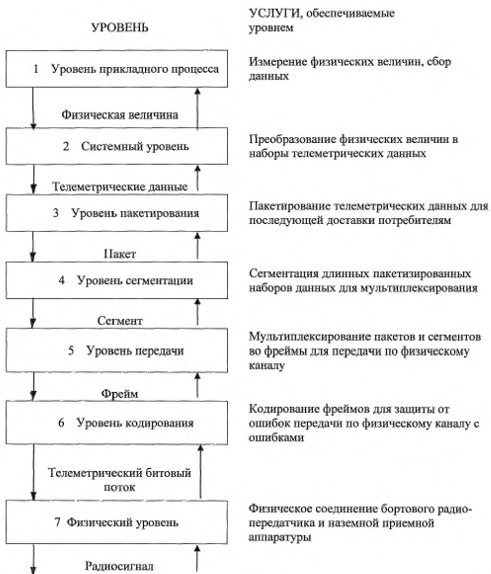
Рисунок 1 — Иерархическая модель телеметрической системы, использующей рекомендации CCSDS
