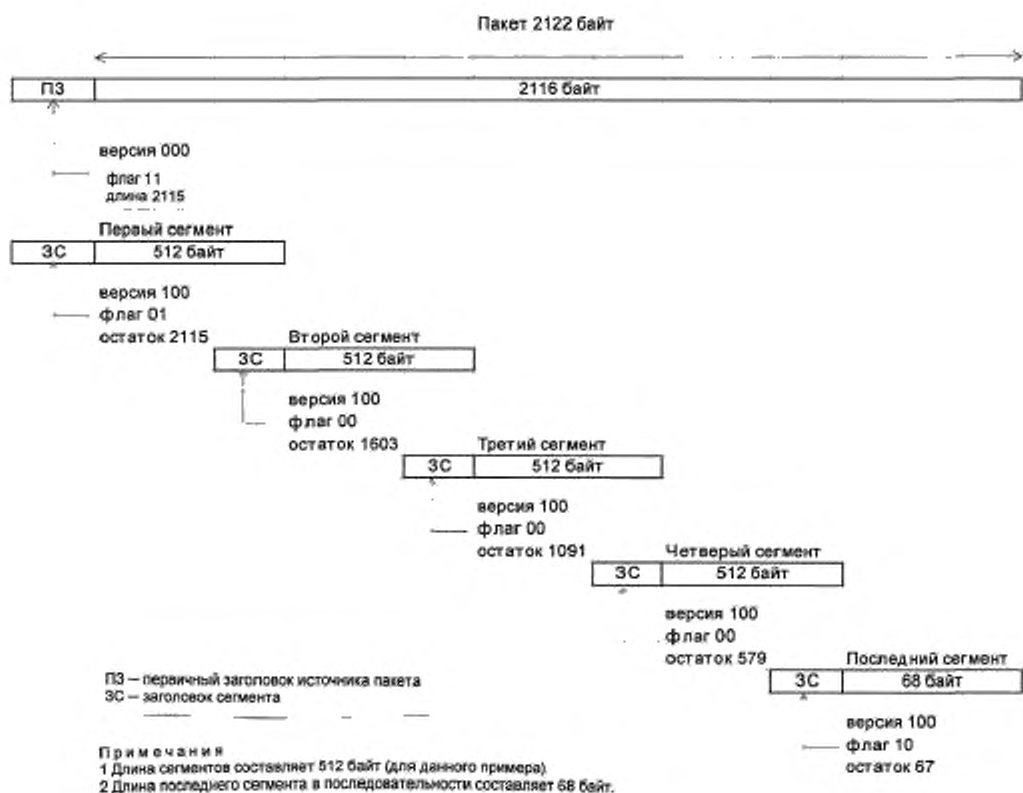
Рисунок 6 – Пример сегментации пакета по источникам данных
