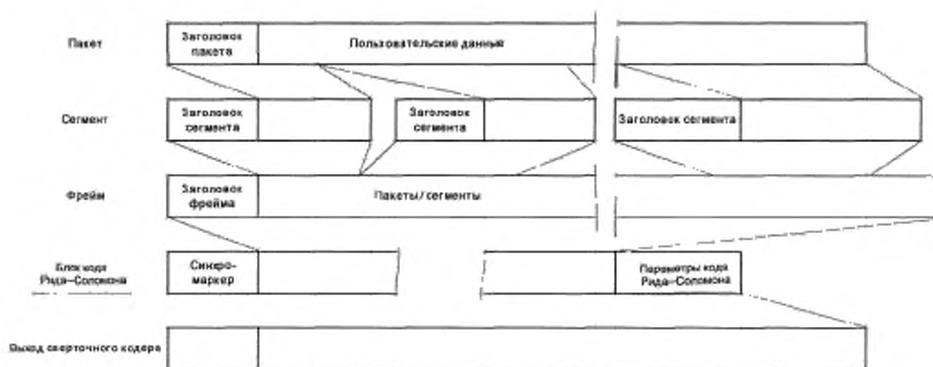
Рисунок 2 — Структуры телеметрических данных
