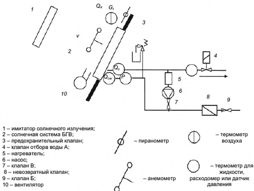
Рисунок В.6 – Схема структуры испытания
