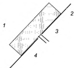
Рисунок В.1 – Солнечная система БГВ, смонтированная на наклонной крыше
