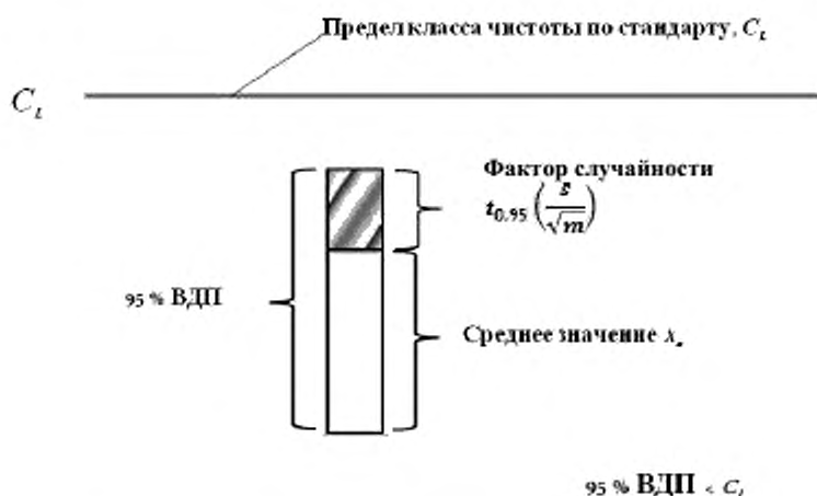
Рисунок А.1 – Графическое представление методики по ГОСТ ИСО 14644-1
