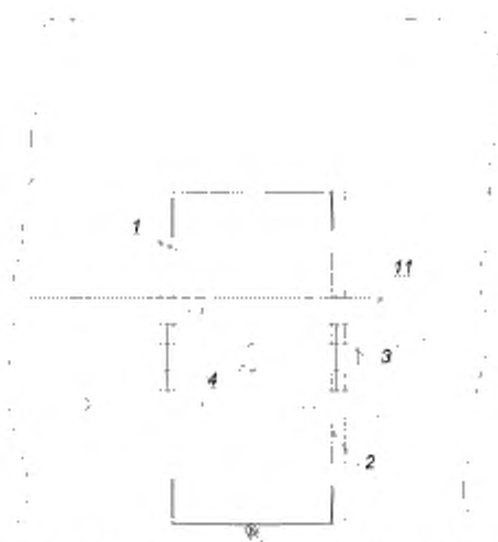
Рисунок 4 – Схема испытания каменной кладки на сцепление
