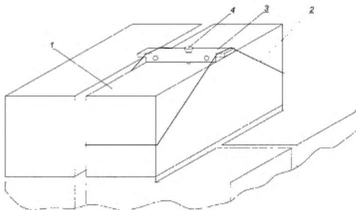
б) схема захвата природного камня
