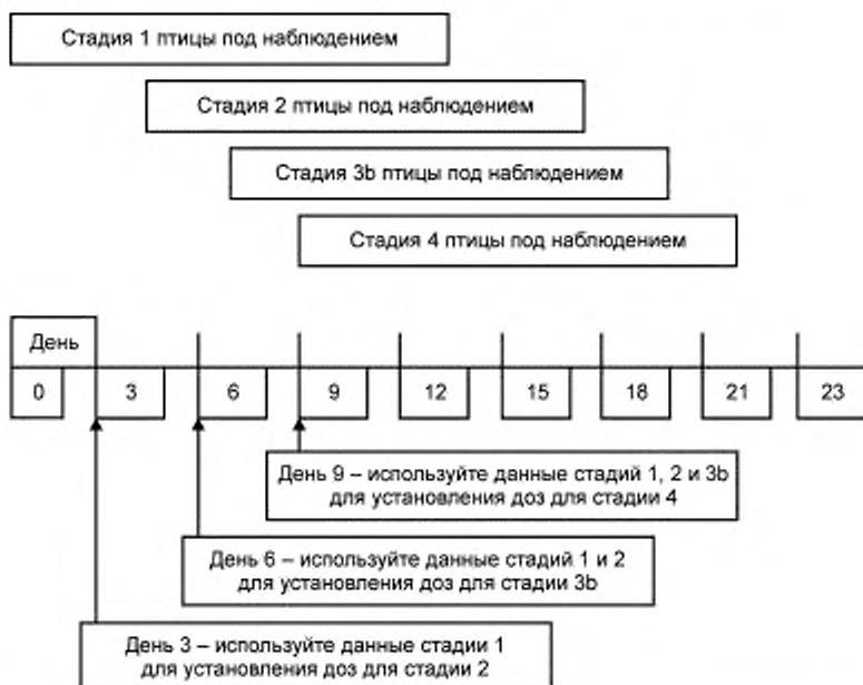
Рисунок 3 — Пример плана-графика последовательной схемы испытания с четырьмя этапами (стадиями 1, 2, 3b и 4) по 14 дней, рисунок не включает контрольную группу птиц
