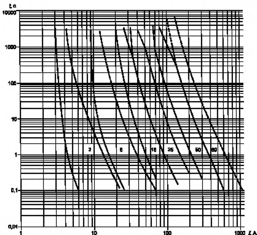
Рисунок А.1 — Время-токовые зоны для плавкого предохранителя
