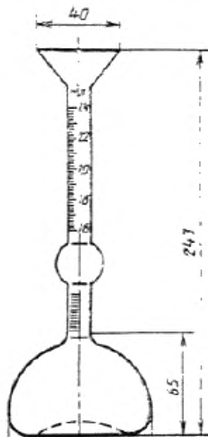
Рисунок 1 — Прибор Ле-Шателье
