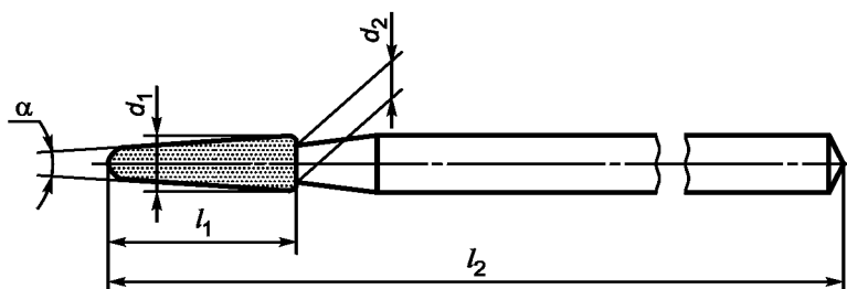
Рисунок 27 — Усеченная коническая с полусферой рабочая часть с длиной головки 6,0 мм
