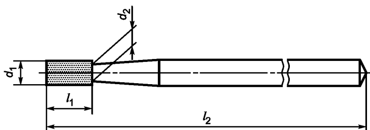
Рисунок 7 — Цилиндрическая рабочая часть с длиной головки 3,0 мм
