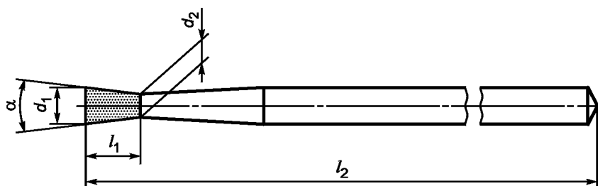
Рисунок 38 — Рабочая часть в виде обратно усеченного конуса с длиной головки 3,5 мм
