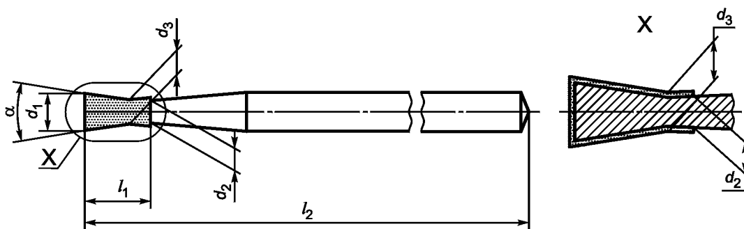
Рисунок 4 — Головка с обратным конусом (с буртиком)
