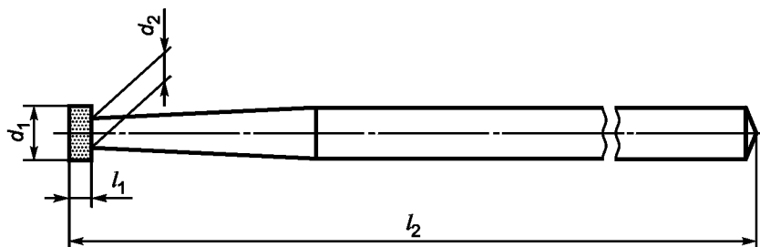
Рисунок 5 — Колесовидная головка
