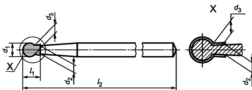
Рисунок 2 — Сферическая головка с буртиком
