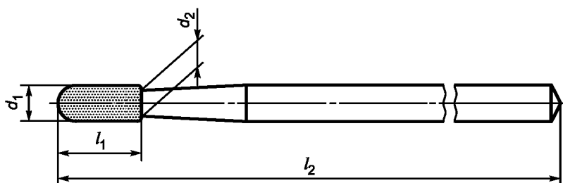
Рисунок 21 — Цилиндрическая полусферическая рабочая часть с длиной головки 4,0 мм
