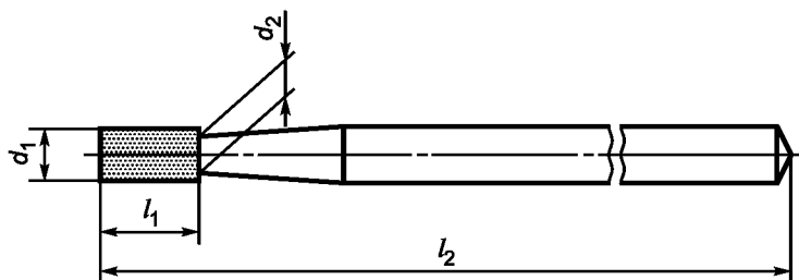
Рисунок 8 — Цилиндрическая рабочая часть с длиной головки 4,0 мм
