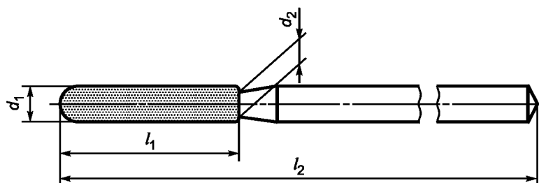
Рисунок 24 — Цилиндрическая полусферическая рабочая часть с длиной головки 9,0 мм
