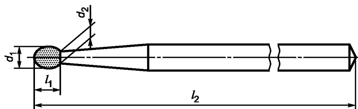
Рисунок 1 — Сферическая головка
