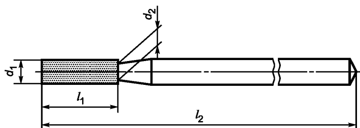
Рисунок 11 — Цилиндрическая рабочая часть с длиной головки 8,0 мм
