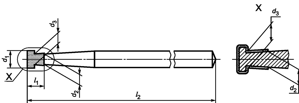
Рисунок 6 — Колесовидная головка с буртиком
