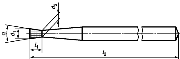
Рисунок 3 — Головка с обратным конусом
